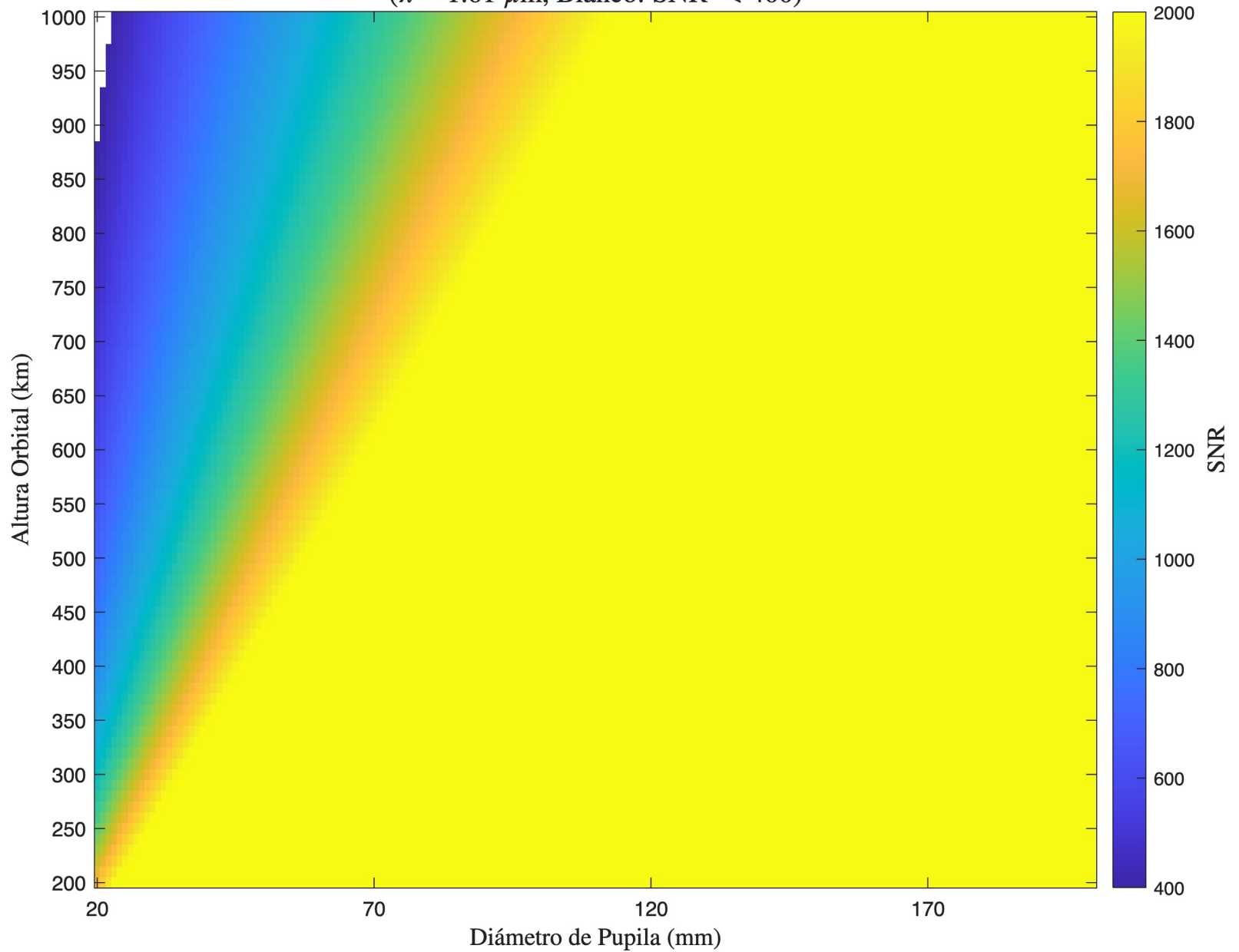
SNR - Cassegrain - Detector 2 ( \lambda = 1.61 \mu\text{m} , Blanco: SNR < 400)
