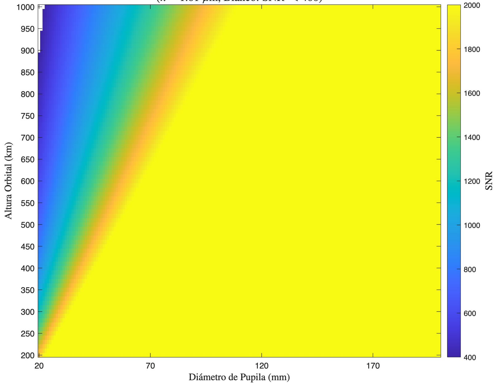
SNR - Refractivo - Detector 3 ( \lambda = 1.61 \mu\text{m} , Blanco: SNR < 400)
