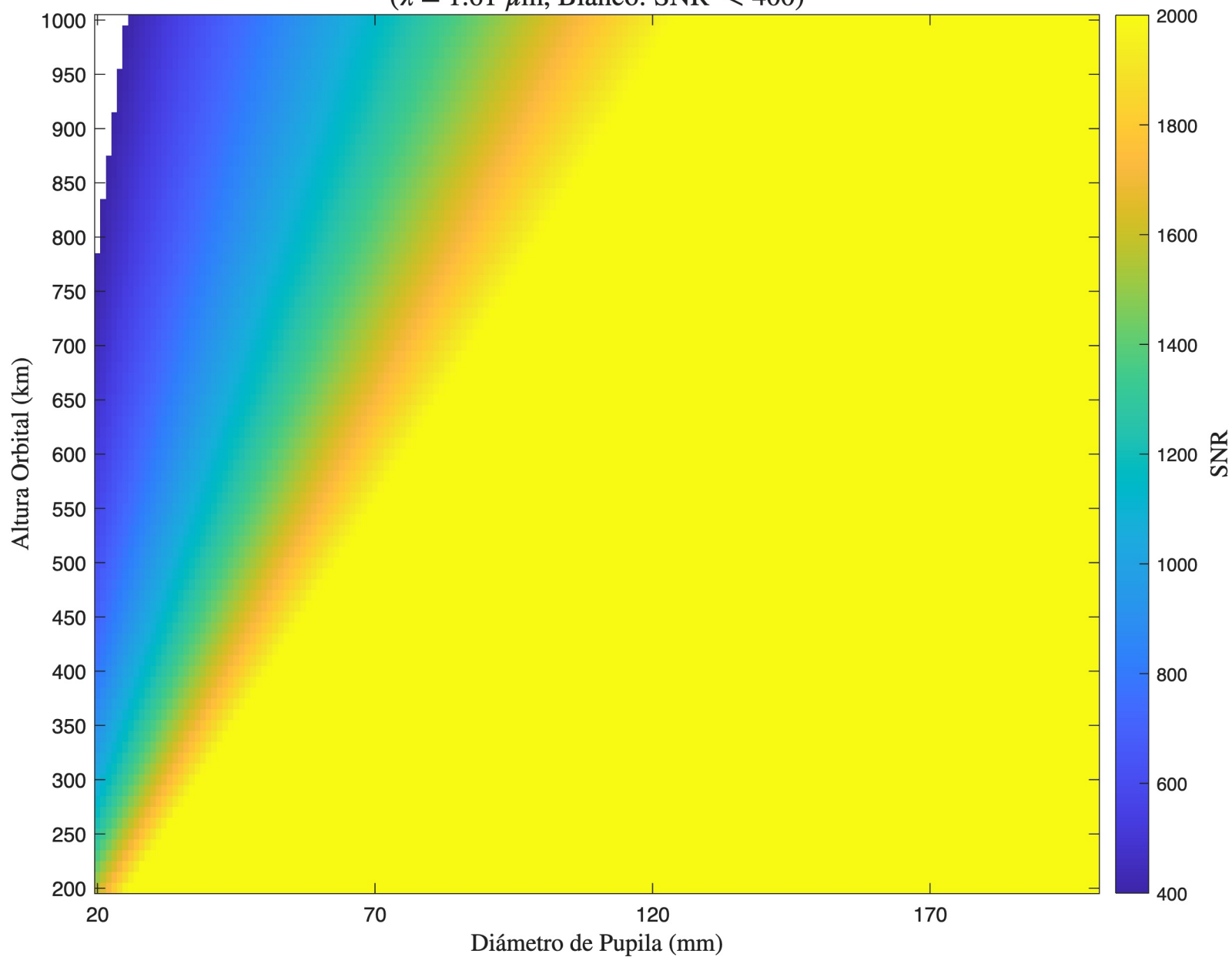
SNR - Korsch - Detector 3 ( \lambda = 1.61 \mu\text{m} , Blanco: SNR < 400)
