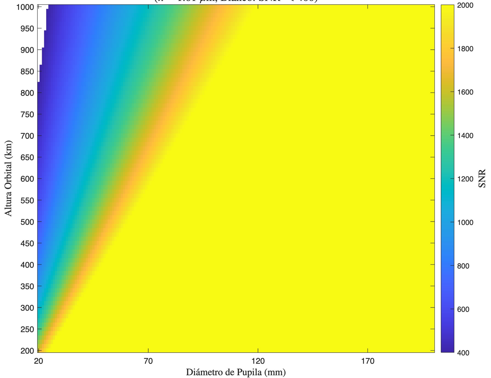
SNR - Cassegrain - Detector 3 ( \lambda = 1.61 \mu\text{m} , Blanco: SNR < 400)
