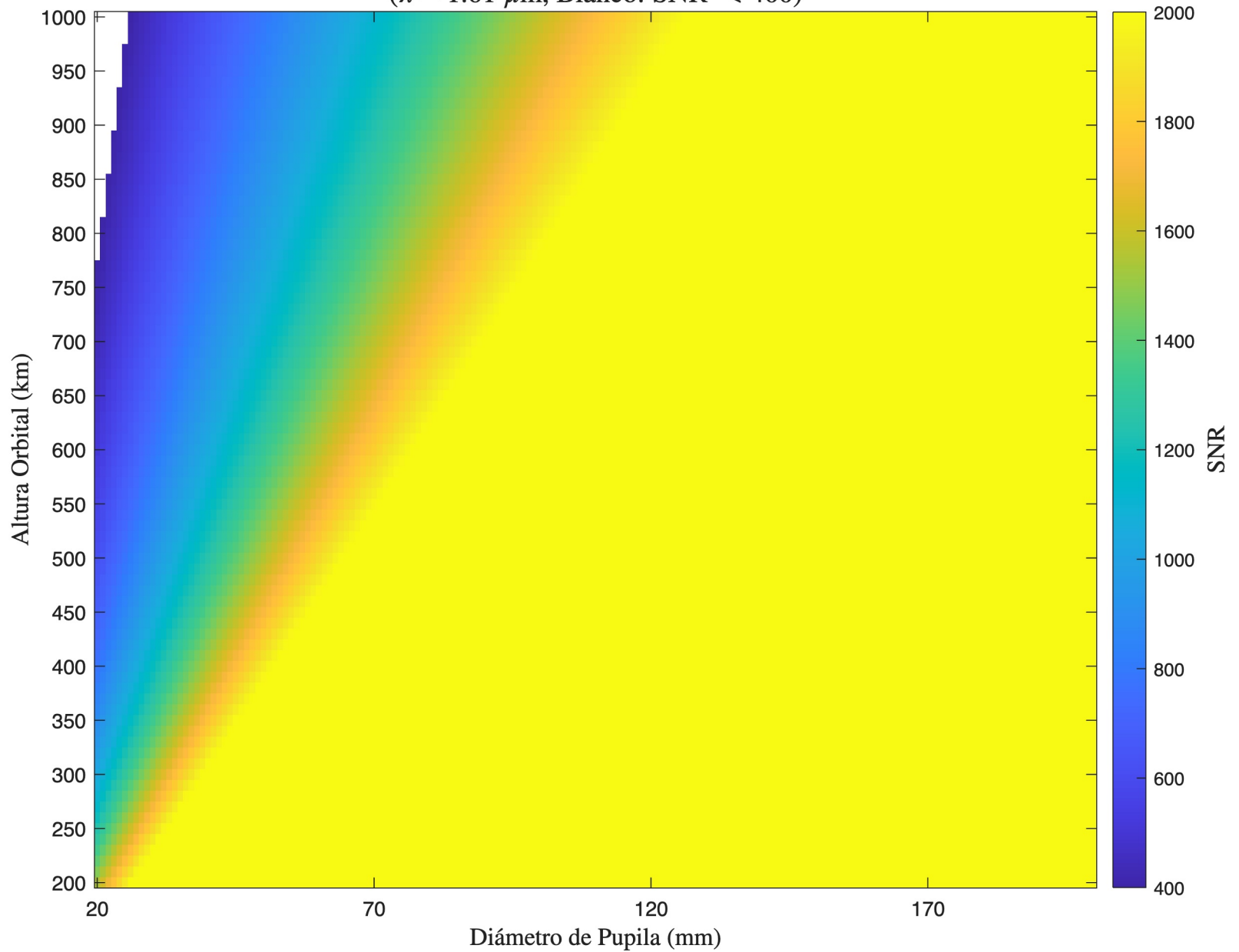
SNR - TMA - Detector 3 ( \lambda = 1.61 \mu\text{m} , Blanco: SNR < 400)
