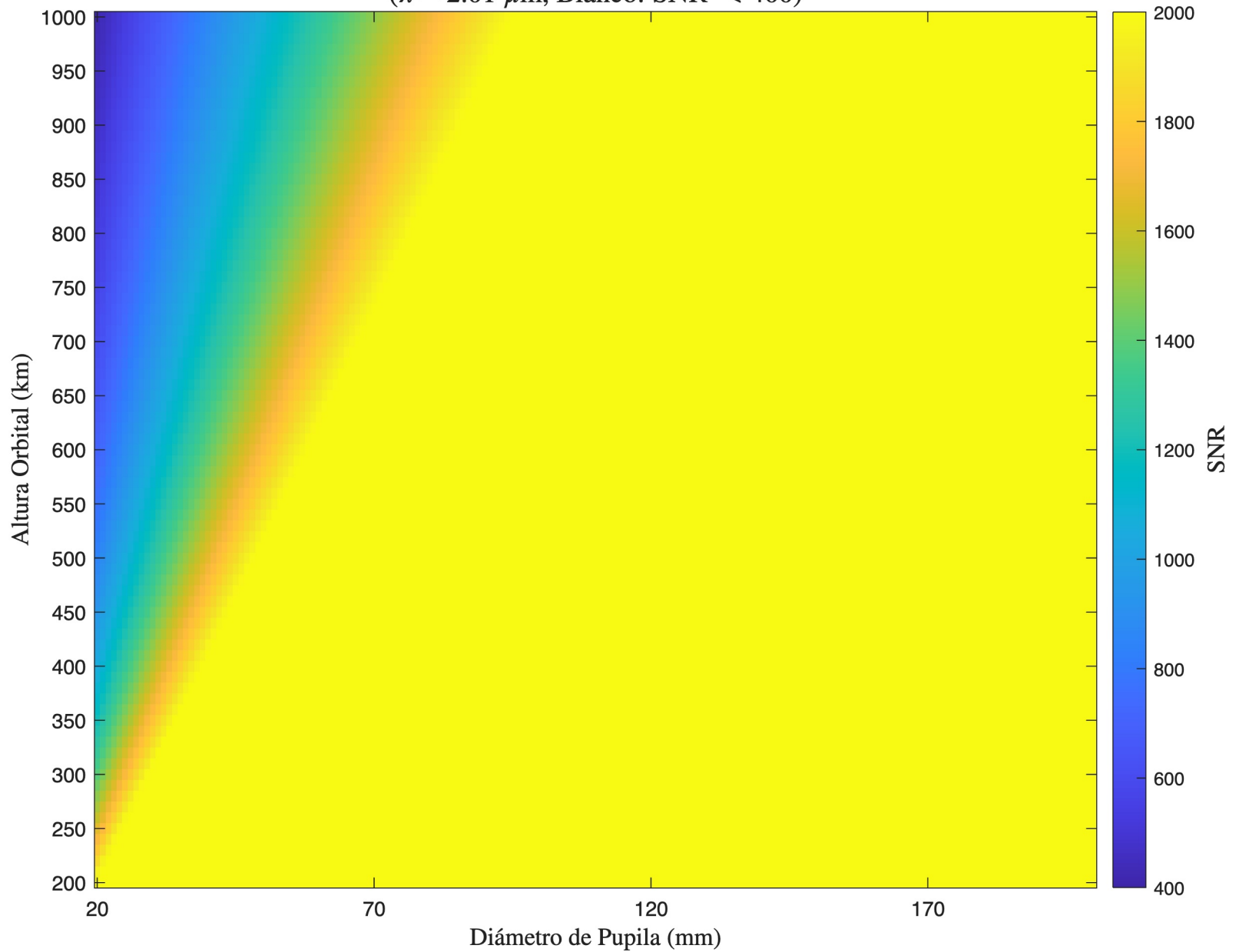
SNR - Korsch - Detector 1 ( \lambda = 2.01 \mu\text{m} , Blanco: SNR < 400)
