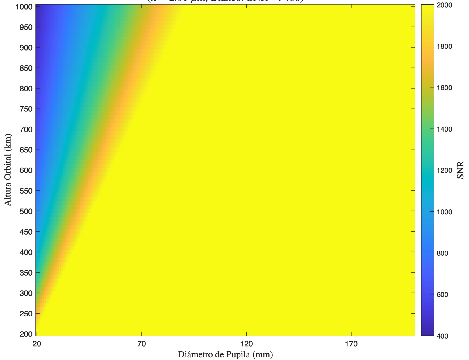
SNR - Cassegrain - Detector 1 ( \lambda = 2.01 \mu\text{m} , Blanco: SNR < 400)
