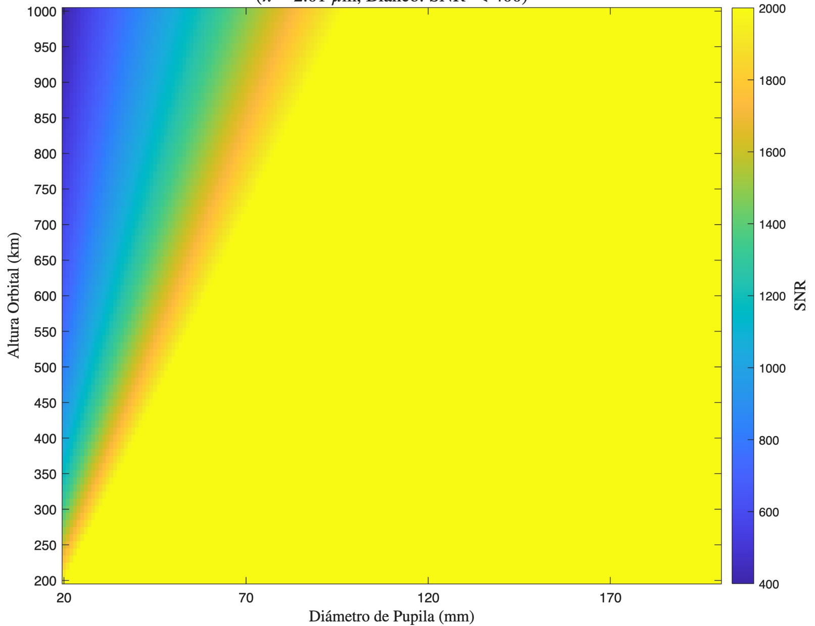
SNR - TMA - Detector 1 ( \lambda = 2.01 \mu\text{m} , Blanco: SNR < 400)
