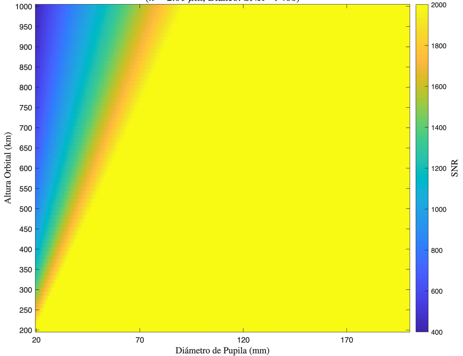
SNR - Refractivo - Detector 2 ( \lambda = 2.01 \mu\text{m} , Blanco: SNR < 400)
