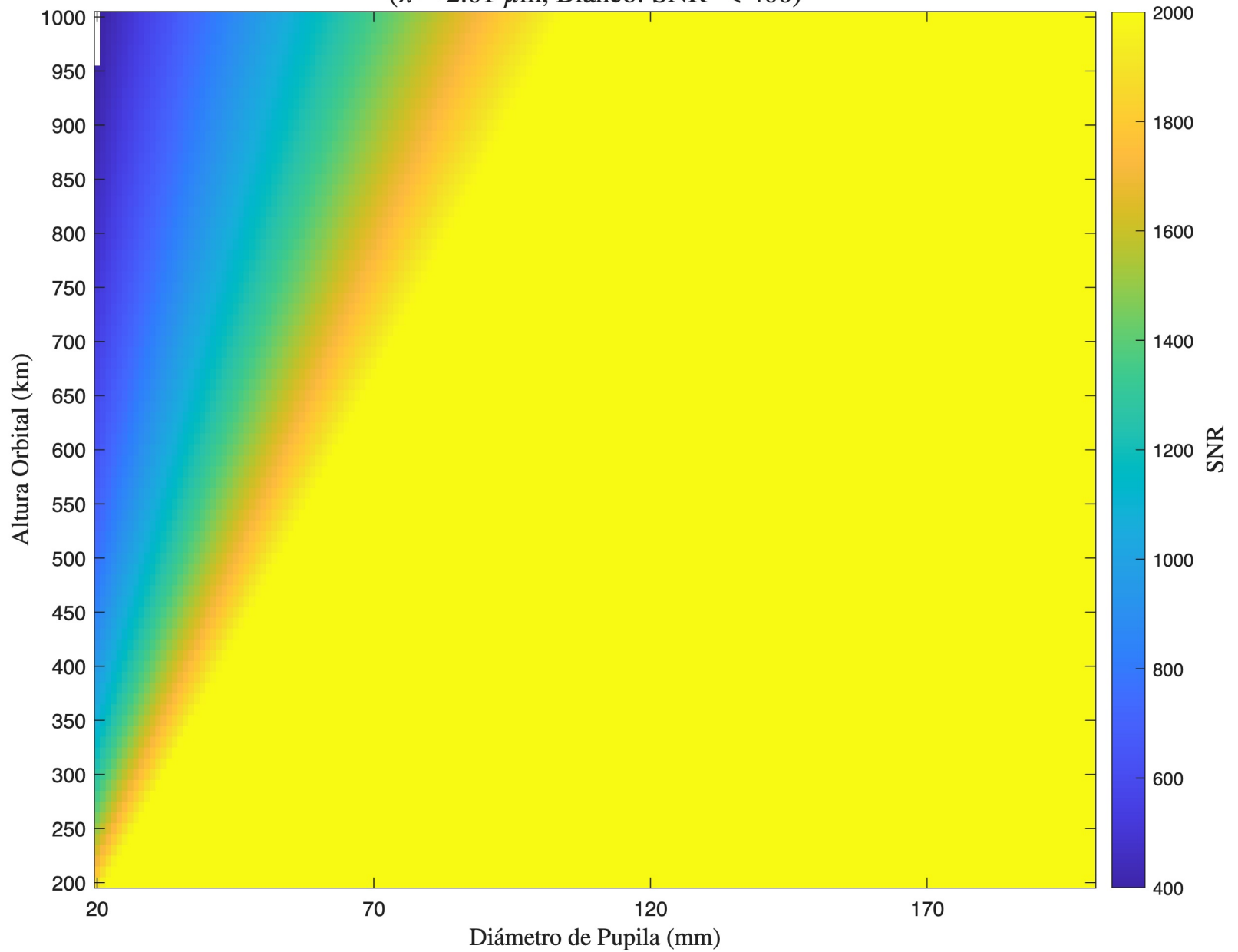
SNR - Korsch - Detector 2 ( \lambda = 2.01 \mu\text{m} , Blanco: SNR < 400)
