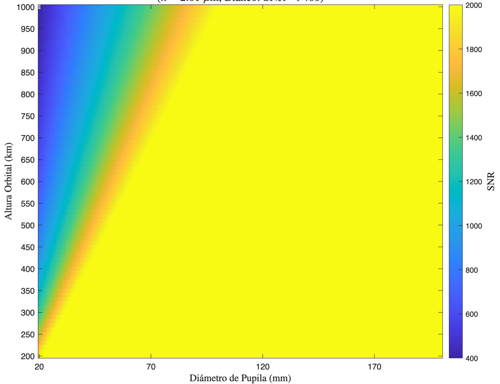
SNR - Cassegrain - Detector 2 ( \lambda = 2.01 \mu\text{m} , Blanco: SNR < 400)
