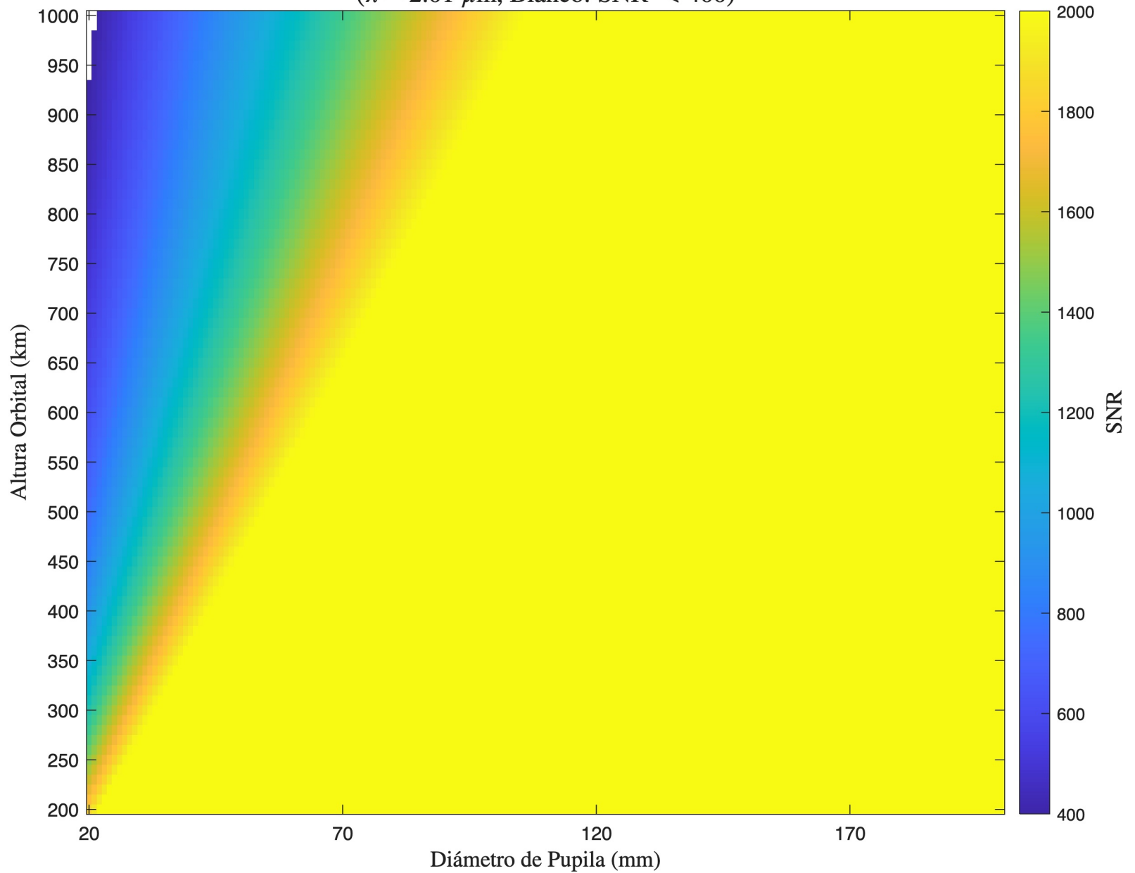
SNR - TMA - Detector 2 ( \lambda = 2.01 \mu\text{m} , Blanco: SNR < 400)
