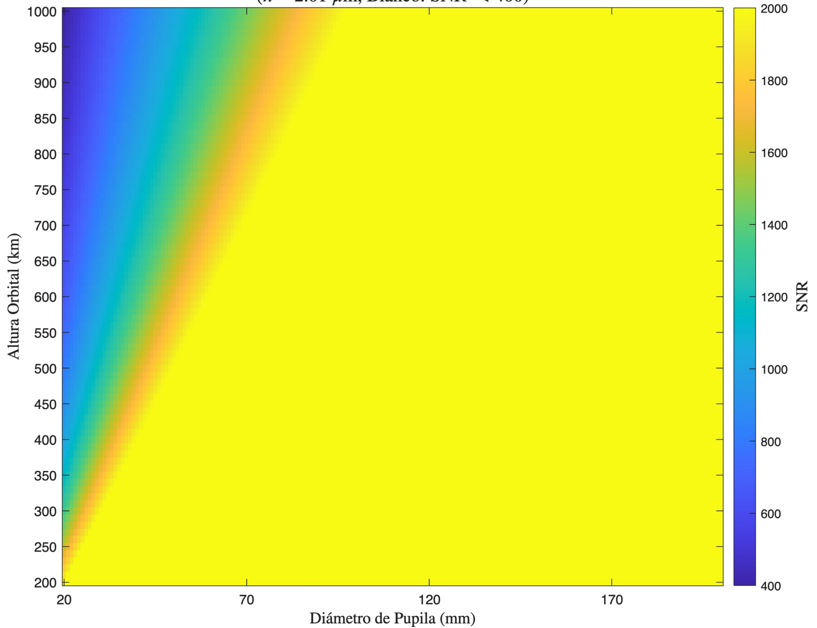
SNR - Refractivo - Detector 3 ( \lambda = 2.01 \mu\text{m} , Blanco: SNR < 400)
