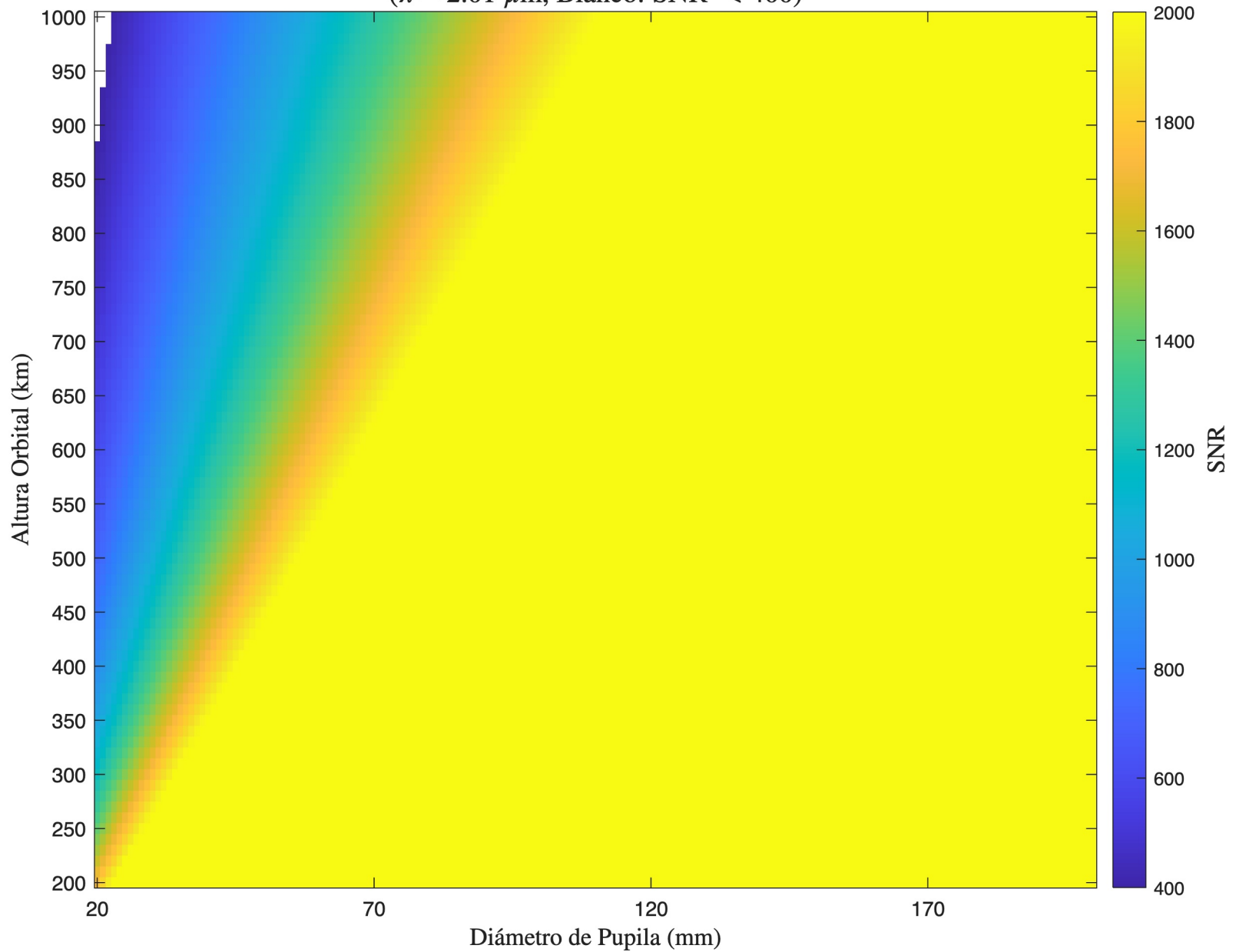
SNR - Korsch - Detector 3 ( \lambda = 2.01 \mu\text{m} , Blanco: SNR < 400)
