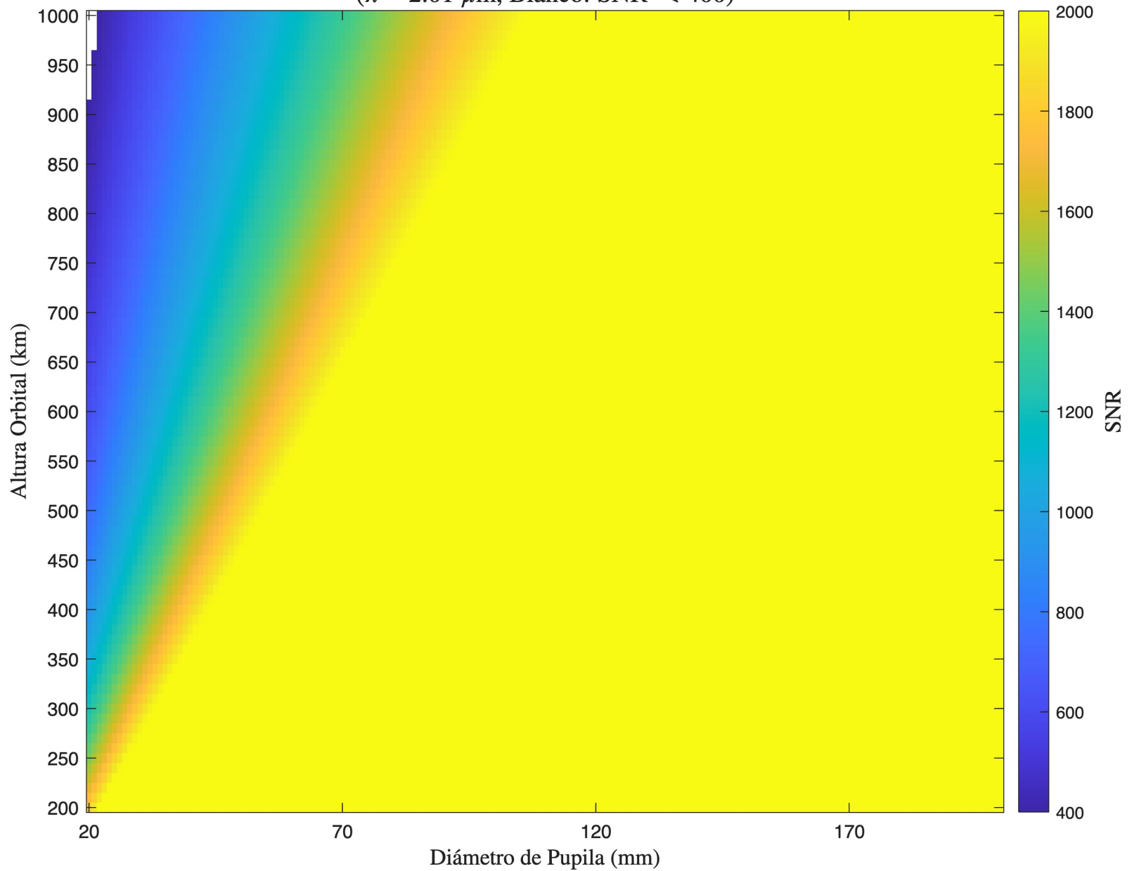
SNR - Cassegrain - Detector 3 ( \lambda = 2.01 \mu\text{m} , Blanco: SNR < 400)
