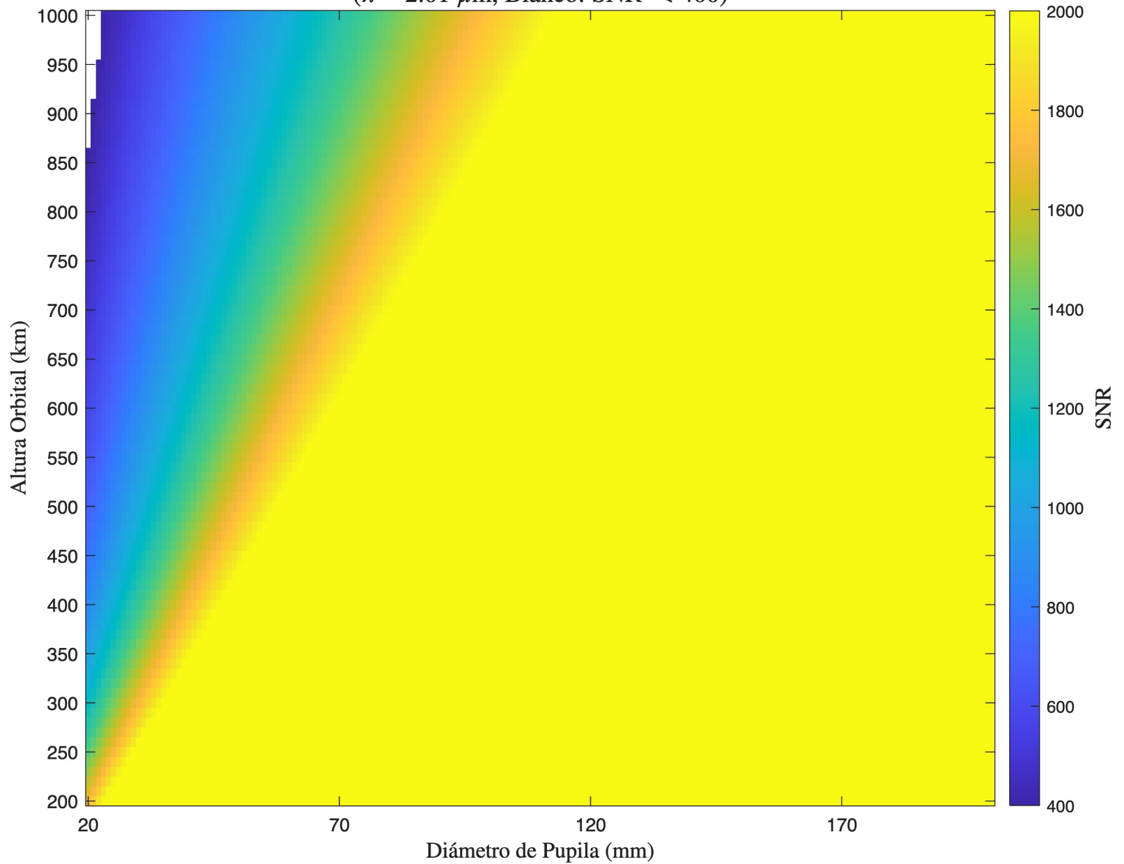
SNR - TMA - Detector 3 ( \lambda = 2.01 \mu\text{m} , Blanco: SNR < 400)
