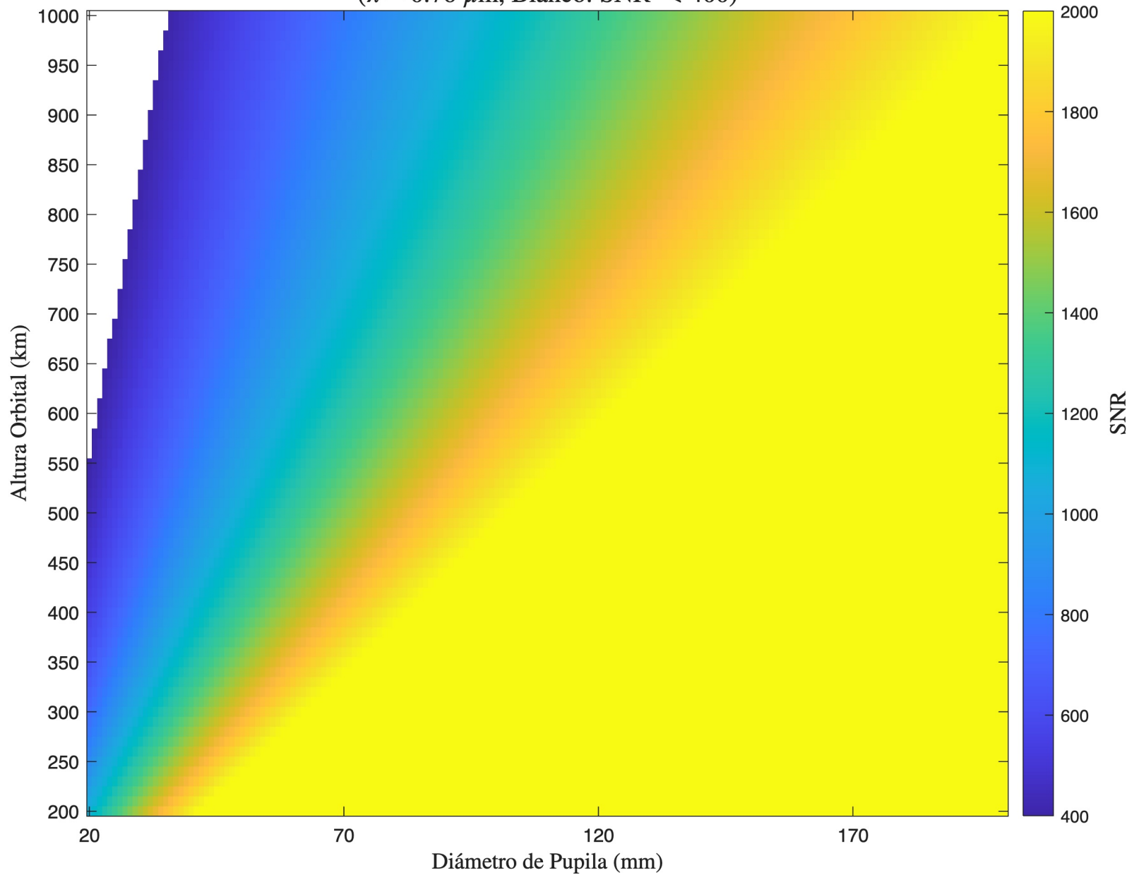
SNR - Korsch - Detector 1 ( \lambda = 0.76 \mu\text{m} , Blanco: SNR < 400)
