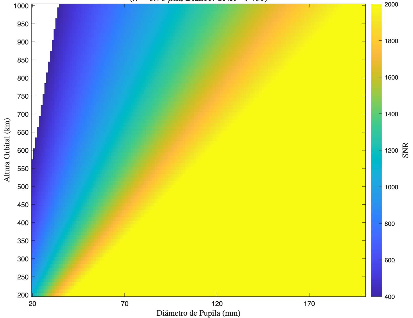
SNR - Cassegrain - Detector 1 ( \lambda = 0.76 \mu\text{m} , Blanco: SNR < 400)
