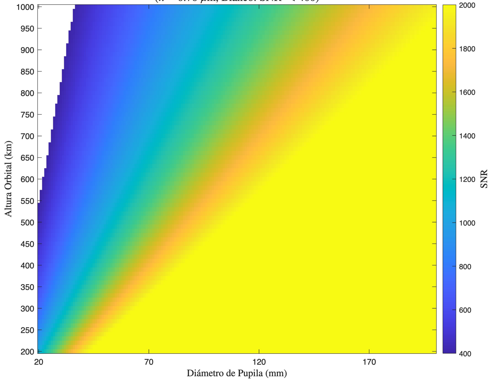
SNR - TMA - Detector 1 ( \lambda = 0.76 \mu\text{m} , Blanco: SNR < 400)
