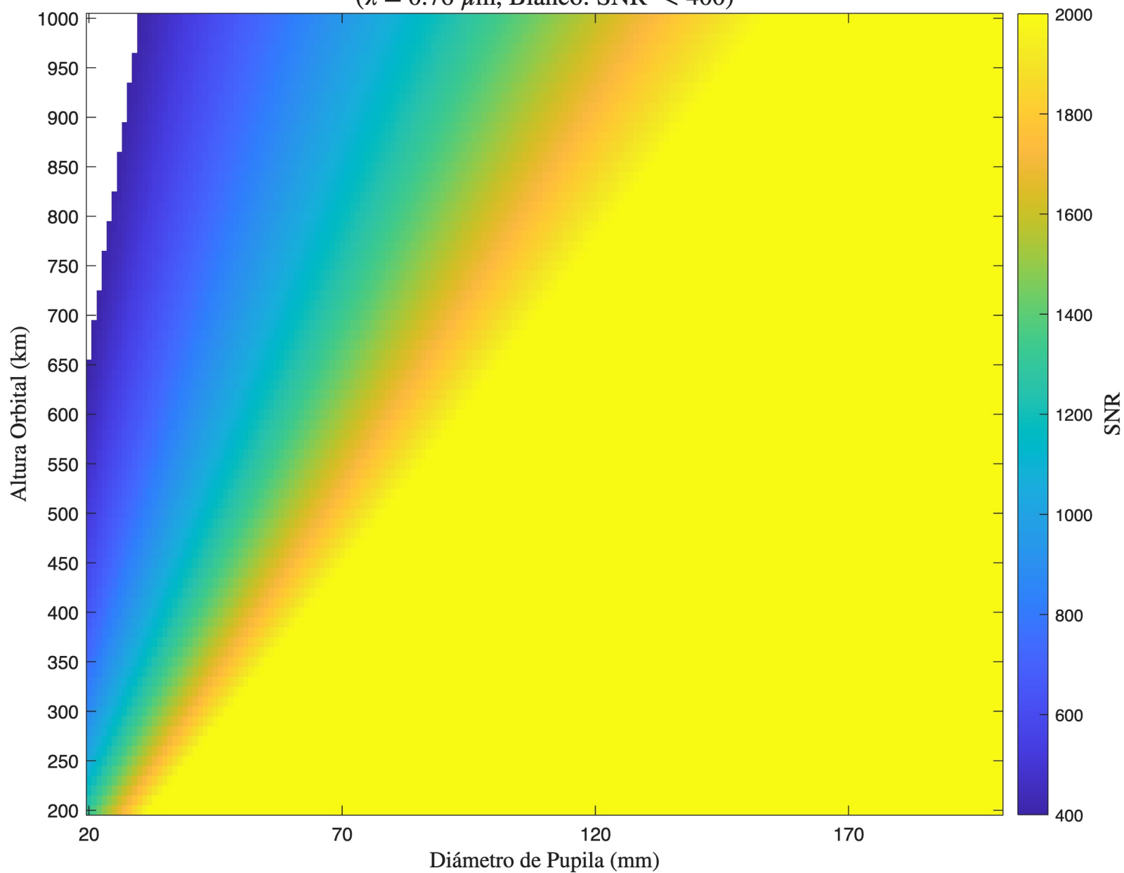
SNR - Refractivo - Detector 2 ( \lambda = 0.76 \mu\text{m} , Blanco: SNR < 400)
