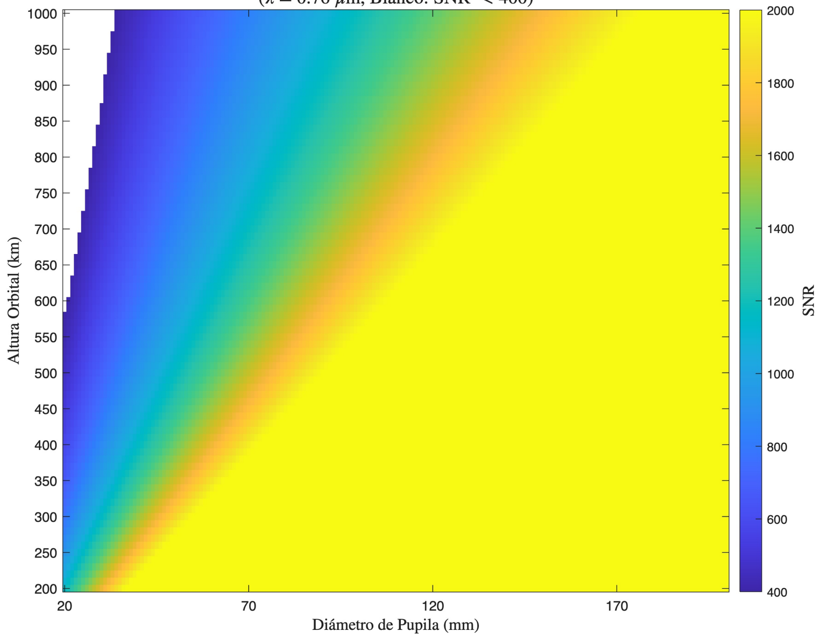
SNR - Korsch - Detector 2 ( \lambda = 0.76 \mu\text{m} , Blanco: SNR < 400)
