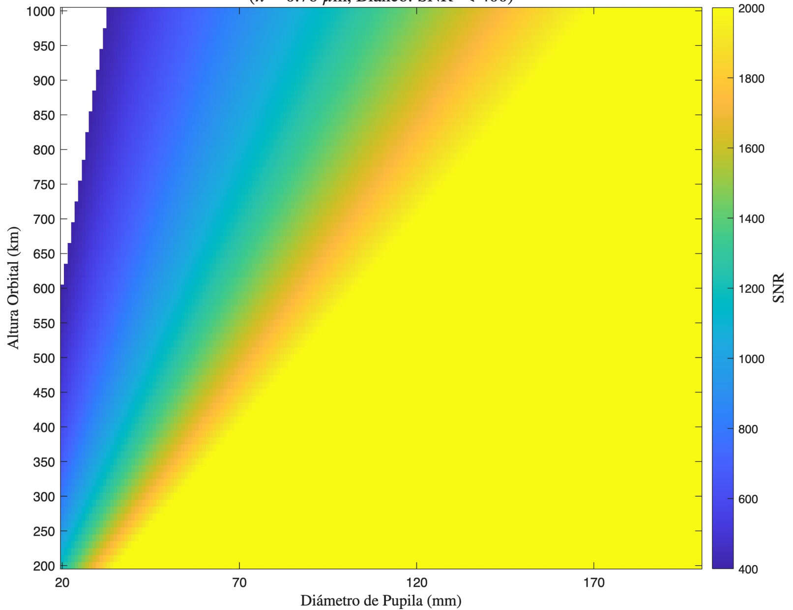
SNR - Cassegrain - Detector 2 ( \lambda = 0.76 \mu\text{m} , Blanco: SNR < 400)
