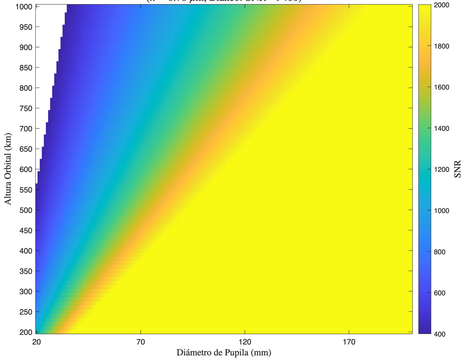
SNR - TMA - Detector 2 ( \lambda = 0.76 \mu\text{m} , Blanco: SNR < 400)
