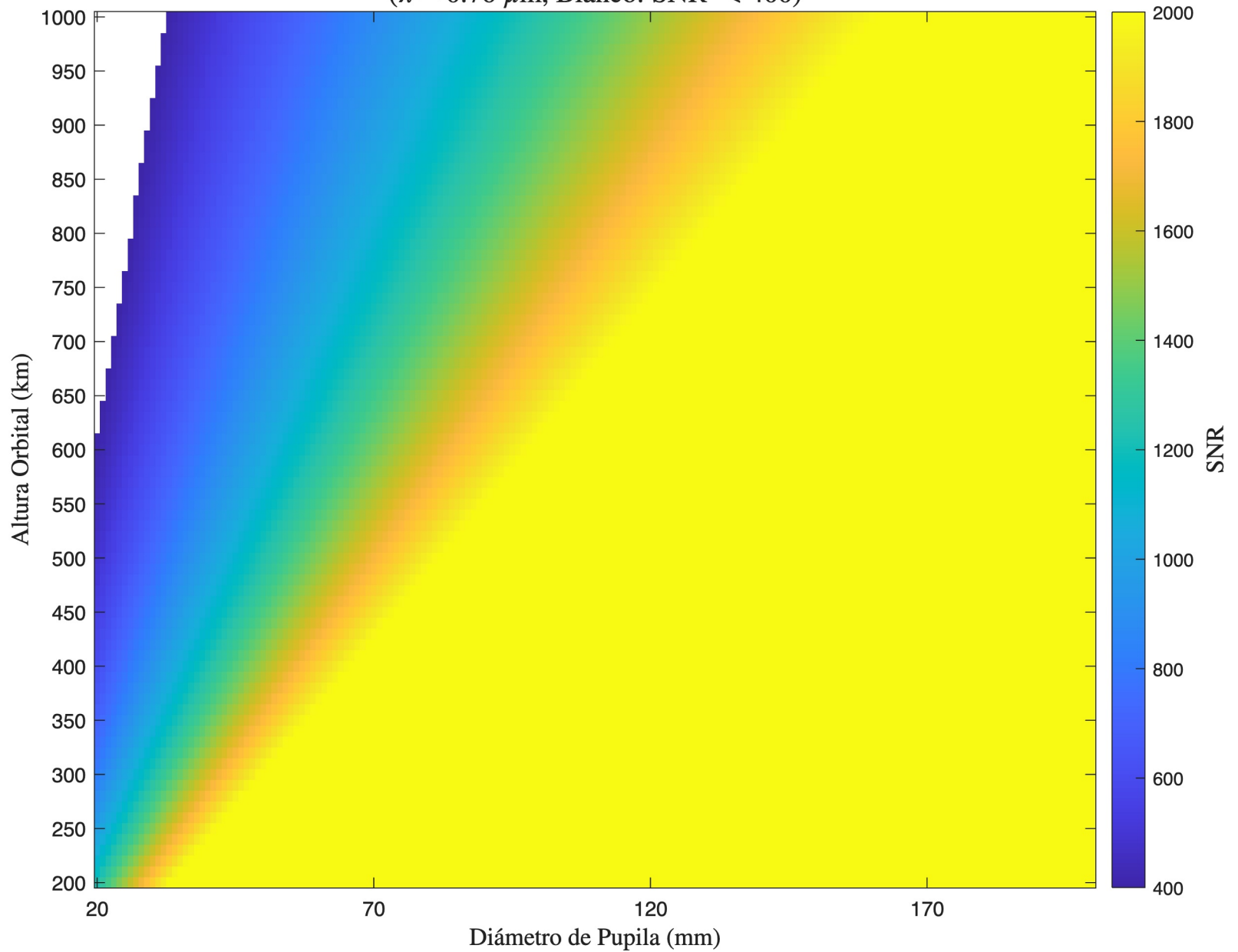
SNR - Refractivo - Detector 3 ( \lambda = 0.76 \mu\text{m} , Blanco: SNR < 400)
