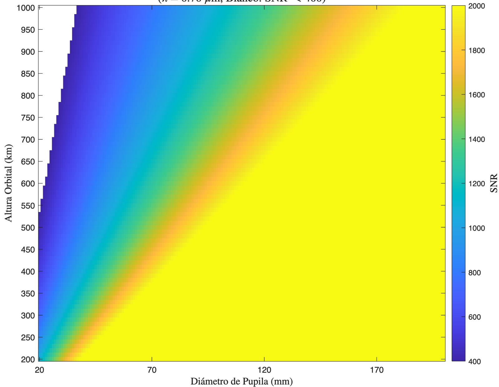
SNR - Korsch - Detector 3 ( \lambda = 0.76 \mu\text{m} , Blanco: SNR < 400)
