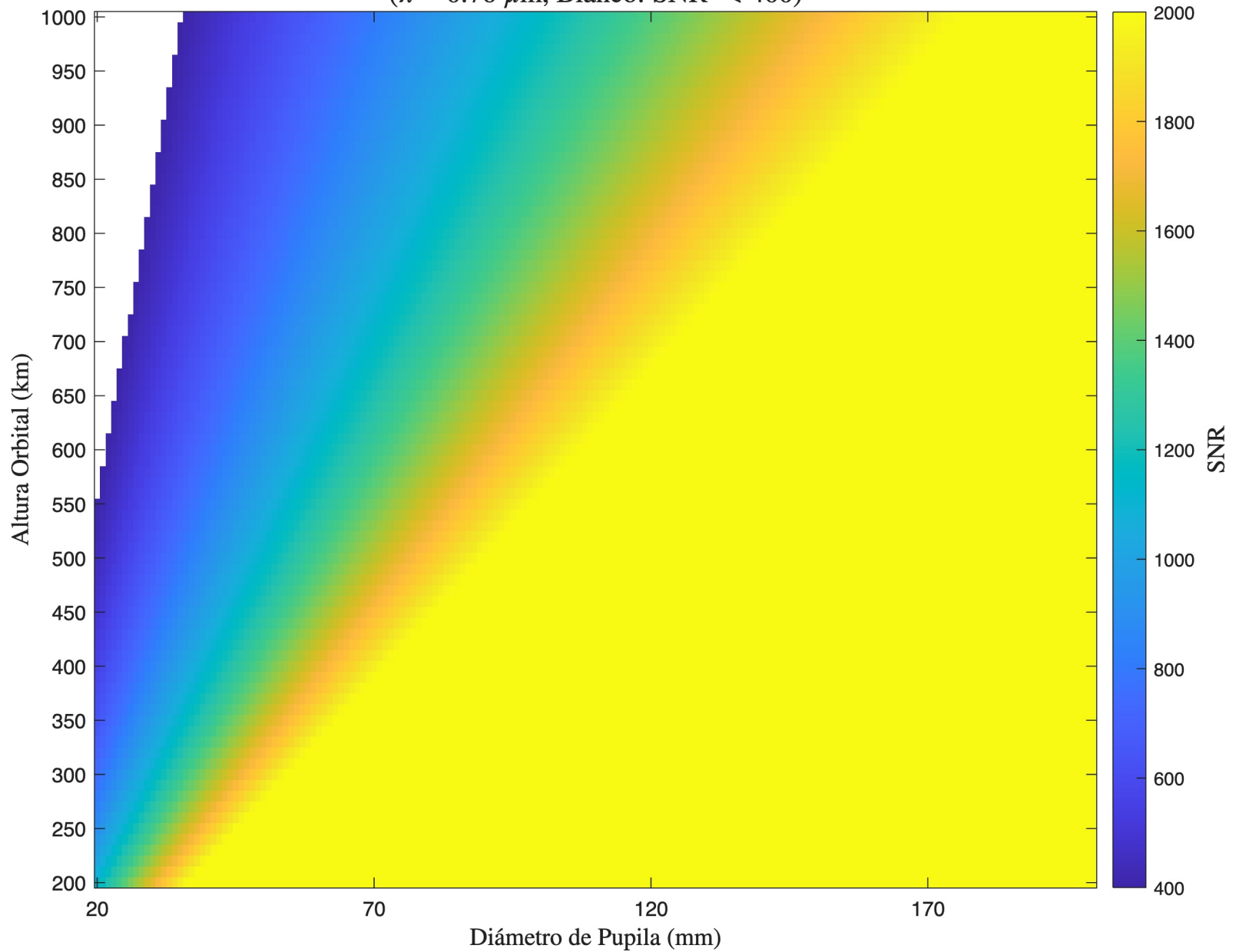
SNR - Cassegrain - Detector 3 ( \lambda = 0.76 \mu\text{m} , Blanco: SNR < 400)
