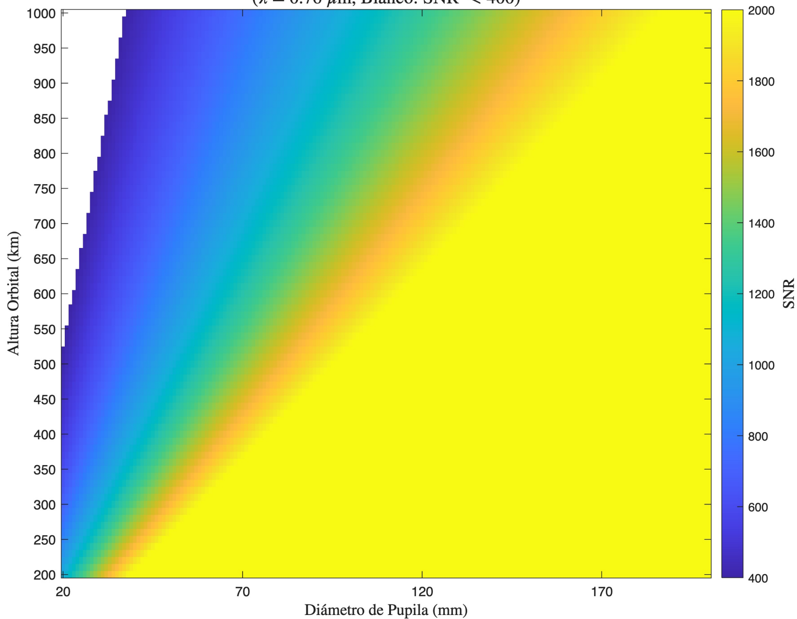
SNR - TMA - Detector 3 ( \lambda = 0.76 \mu\text{m} , Blanco: SNR < 400)
