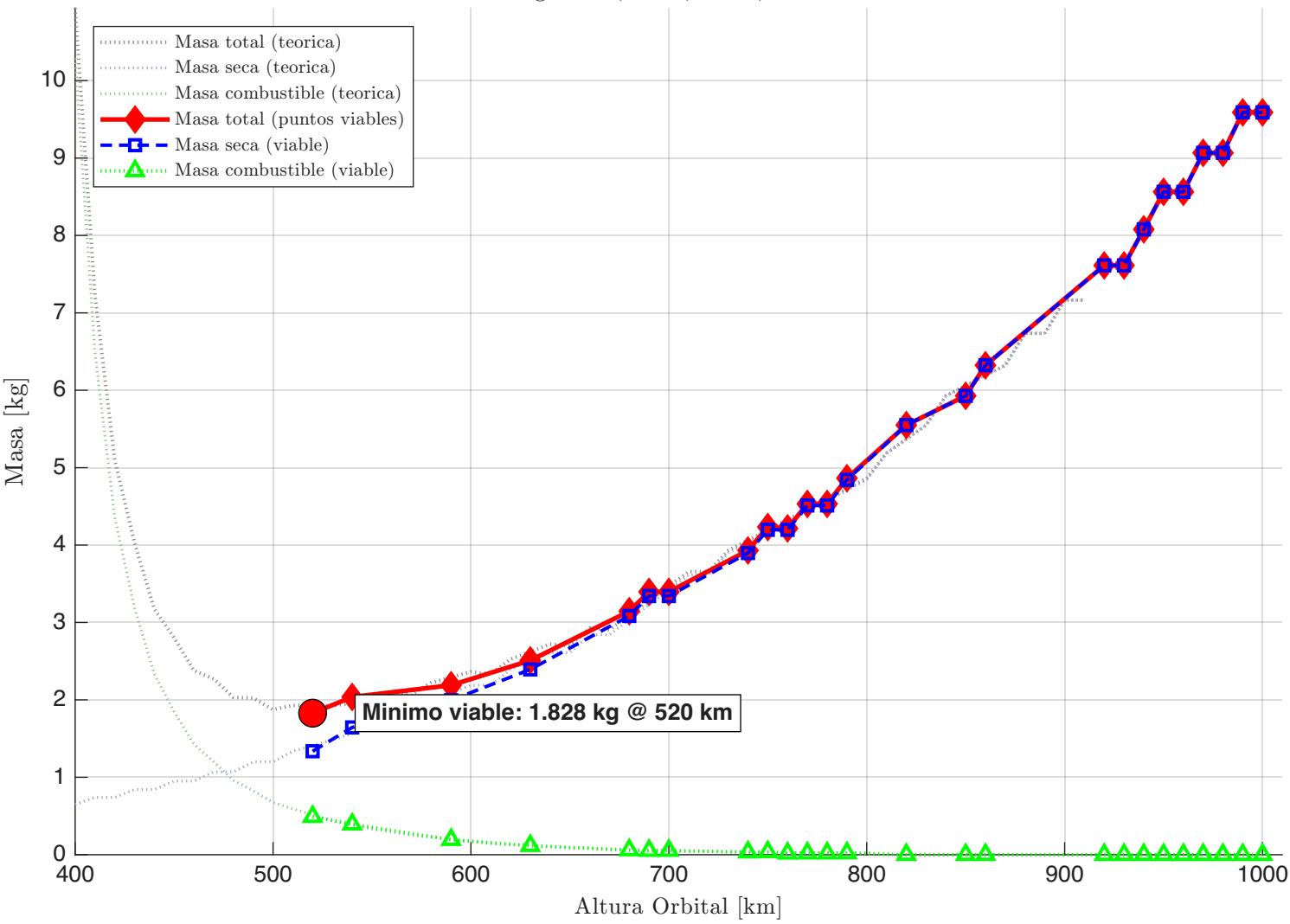
Desglose de Masas vs. Altura Config: 2 Sat, 2 Tel, Det 2, Refractivo
