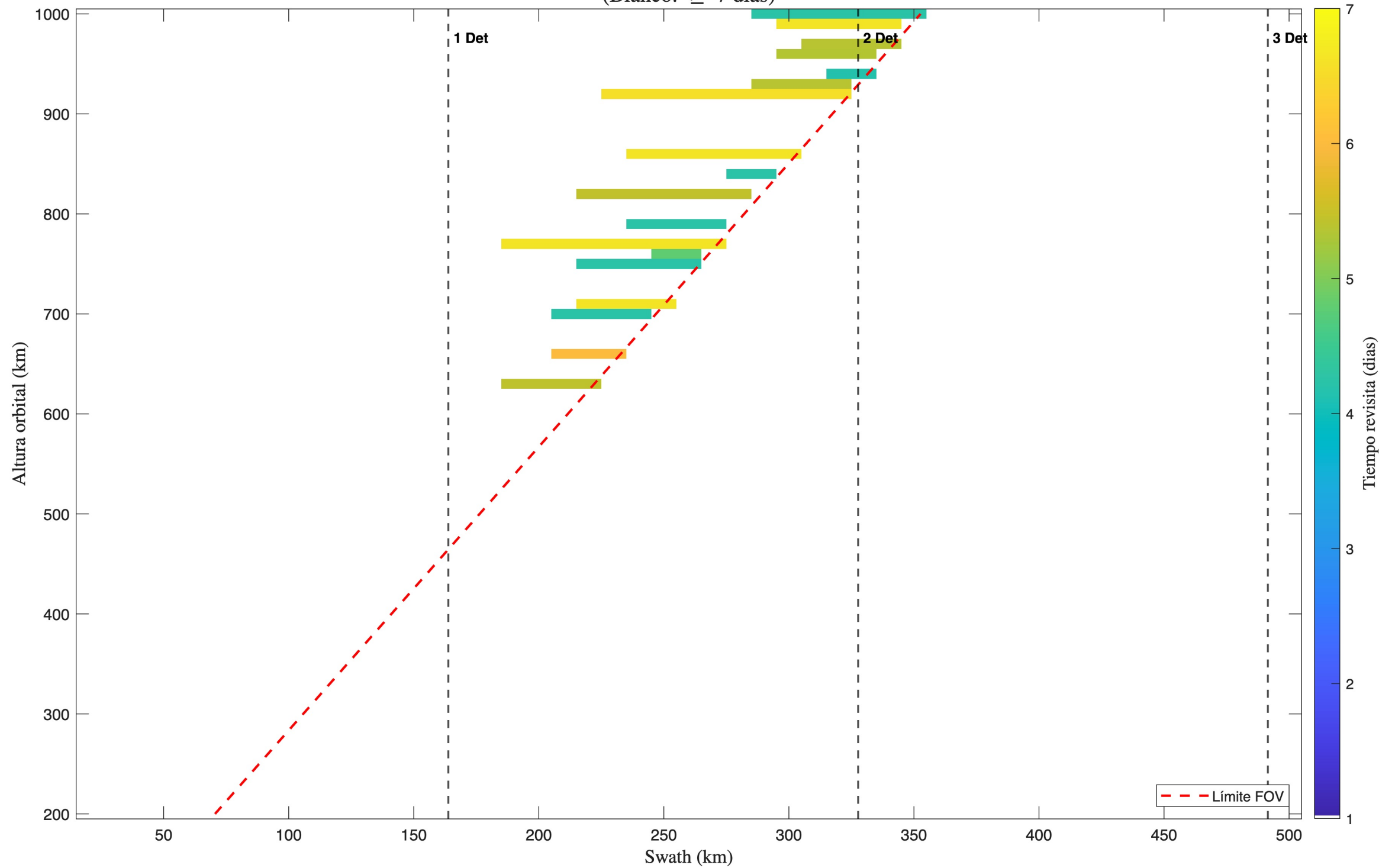
Tiempo Revisita - 2 Satellite(s); 2 Telescopio(s): Refractivo; Detector 2 (Blanco: \geq 7 días)
