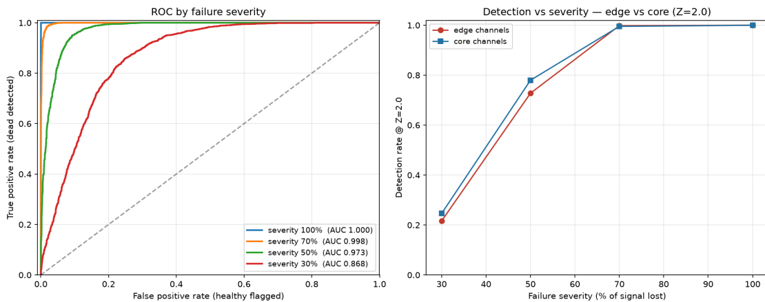
Figura 1.6: Validación del estadístico de detección mediante inyección de fallos con verdad conocida. Izquierda: curvas ROC para distintas severidades. Derecha: tasa de detección en el punto de operación, desglosada entre canales de borde y centrales.
