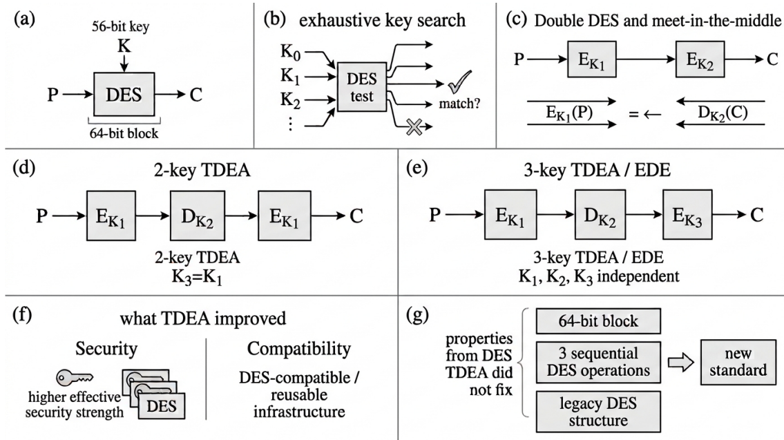
Slika 2: Od DES-a ka TDEA kao tranzicionom rešenju. Panel (a) prikazuje osnovne parametre DES-a, dok (b) ilustruje praktični značaj ograničenog 56-bitnog prostora ključeva. Panel (c) prikazuje Double DES i princip meet-in-the-middle napada. Paneli (d) i (e) prikazuju dvo- i troključnu TDEA EDE konstrukciju. Panel (f) sažima glavne tranzicione prednosti TDEA: veću sigurnosnu snagu i mogućnost ponovne upotrebe postojeće DES infrastrukture. Panel (g) prikazuje ograničenja koja TDEA nije uklonio, pre svega 64-bitni blok, trošak tri sekvencijalne DES operacije i nasleđenu strukturu DES-a.
