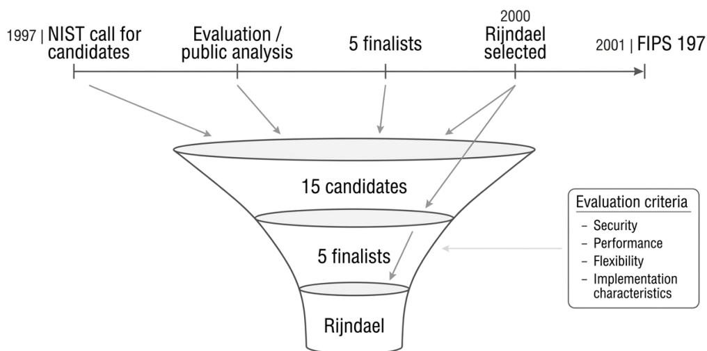
Slika 3: Proces izbora AES-a prikazan kao kombinacija vremenske linije i sužavanja skupa kandidata. NIST je 1997. godine objavio poziv za kandidate, nakon čega je razmatrano 15 predloženih algoritama. Evaluacija je obuhvatila bezbednost, performanse, fleksibilnost i implementacione karakteristike, što je dovelo do izdvajanja pet finalista, izbora Rijndaela 2000. godine i njegovog usvajanja kao standarda FIPS 197 2001. godine.
