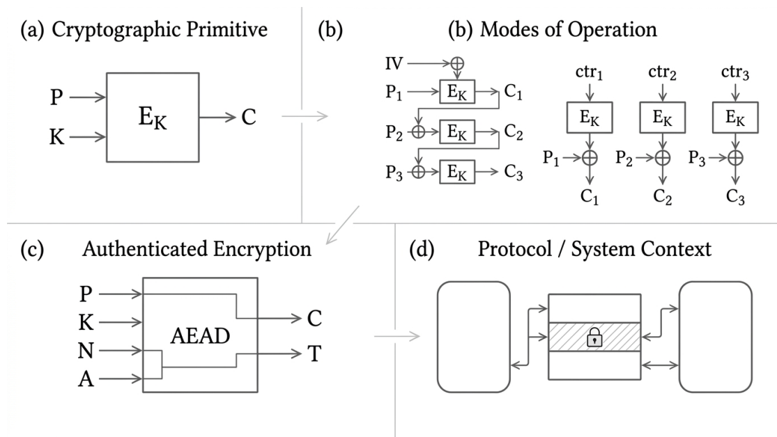
Slika 1: Hijerarhija apstrakcije u simetričnoj kriptografiji. Panel (a) prikazuje blokovsku šifru kao osnovnu kriptografsku primitivu, panel (b) način na koji se ista primitiva koristi kroz modove rada nad više blokova, panel (c) proširenje ka autentifikovanoj enkripciji sa zaštitom poverljivosti i integriteta, a panel (d) ugradnju takvih mehanizama u širi protokolski ili sistemski kontekst. Slika je namerno svedena na strukturne odnose; terminološka i funkcionalna objašnjenja data su u tekstu.
