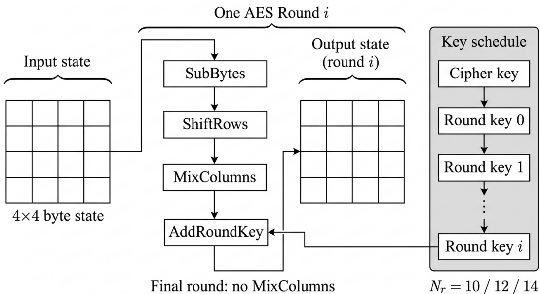
Slika 4: Shematski prikaz strukture jednog tipičnog AES kruga i rasporeda ključeva. Ulazno stanje organizovano je kao matrica od 4 \times 4 bajta, nad kojom se redom primenjuju transformacije SubBytes , ShiftRows , MixColumns i AddRoundKey . Zasebni key schedule iz glavnog ključa generiše rundne ključeve koji se koriste u koraku AddRoundKey . Završni krug izostavlja MixColumns , dok broj krugova zavisi od dužine ključa i iznosi N_r = 10, 12 ili 14 za AES-128, AES-192 i AES-256.
