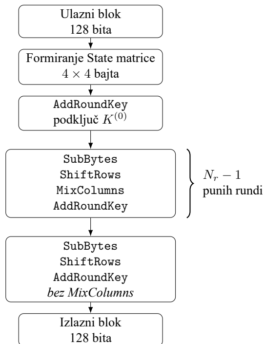
Slika 5: Tok AES šifrovanja. Nakon početnog AddRoundKey koraka izvršava se N_r - 1 punih rundi, dok završna runda ne sadrži MixColumns. Broj rundi iznosi 10, 12 ili 14 za AES-128, AES-192 odnosno AES-256.
