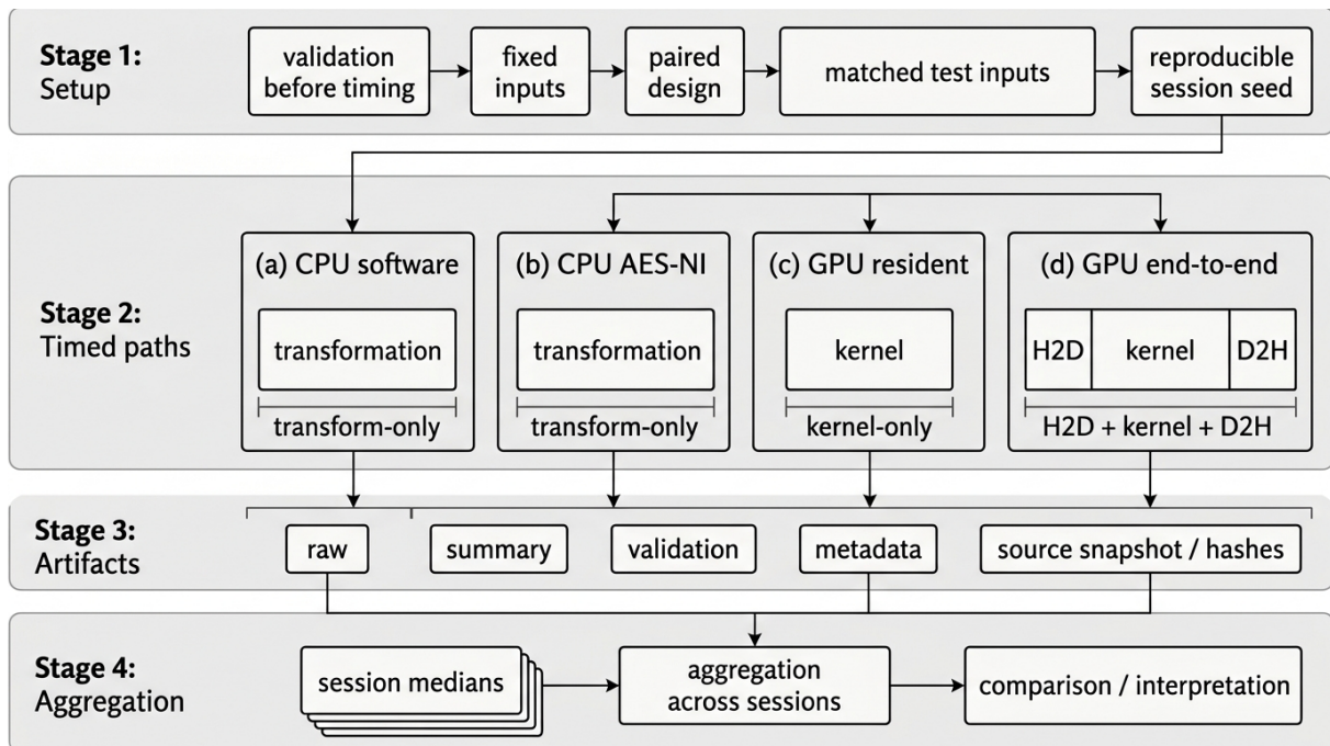
Slika 7: Metodološki okvir eksperimentalne analize. Figura prikazuje sled od validacije i pripreme uparenih ulaza, preko četiri merene izvršne putanje, do čuvanja eksperimentalnih artefakata i završne agregacije rezultata kroz više nezavisnih sesija. Posebno su izdvojene granice merenja za CPU putanje ( transform-only ), GPU resident putanju ( kernel-only ) i GPU end-to-end putanju ( H2D + kernel + D2H ). Time se eksplicitno razdvajaju korektnost, opseg merenja i naknadna interpretacija rezultata.
