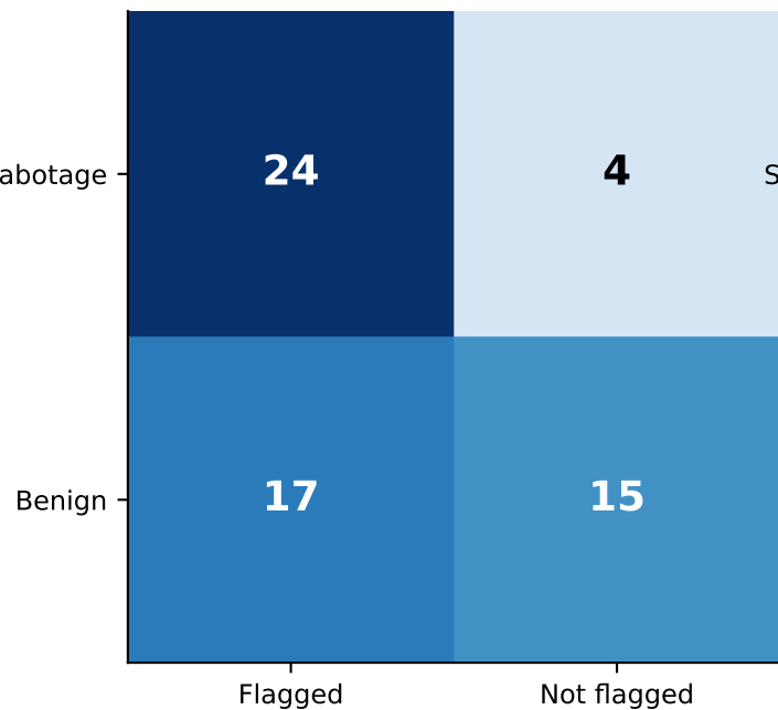
Allam-2-7B
