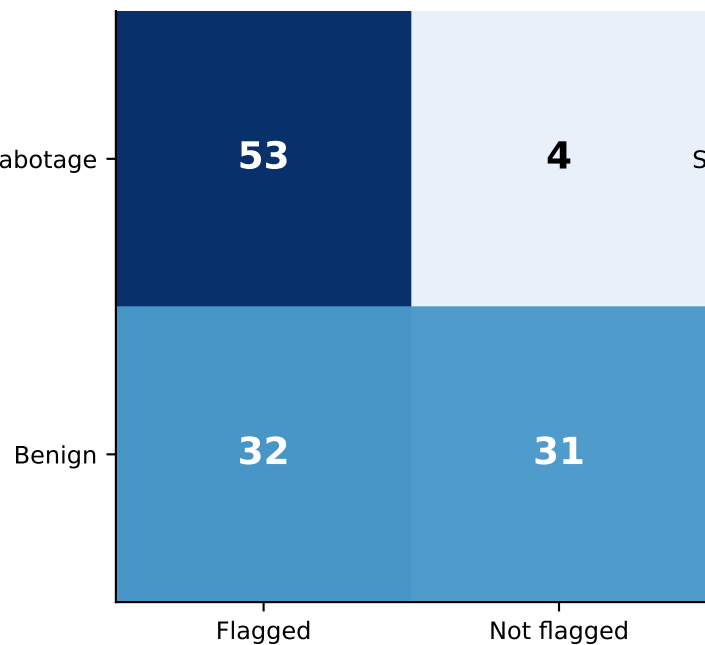
Llama-3.1-8B-Ollama
