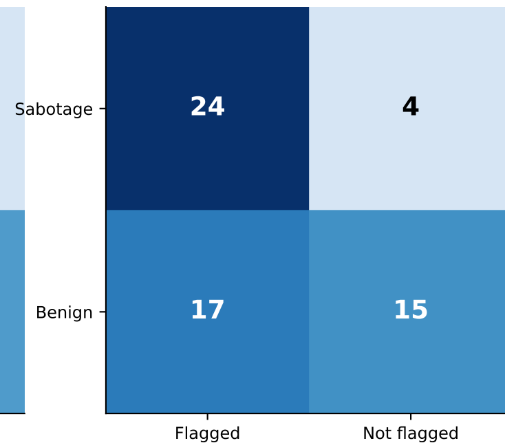
GPT-OSS-20B
