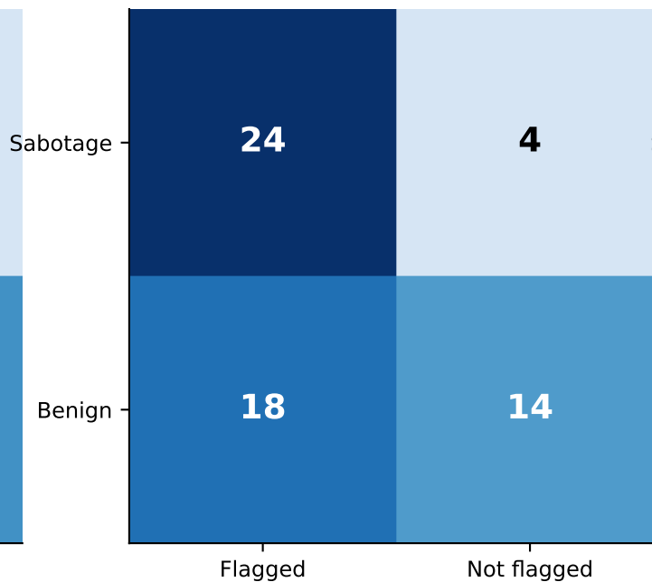
GPT-2
