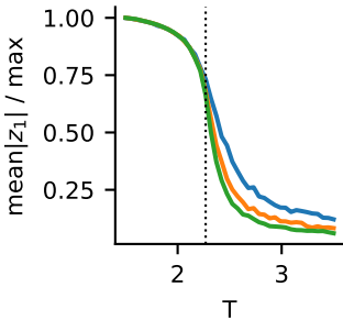
PCA
