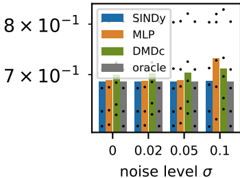
Van der Pol
