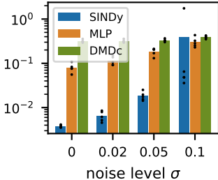
Van der Pol
