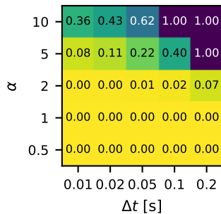
DT-CBF (DI)
