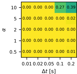
CT-CBF (DI)
