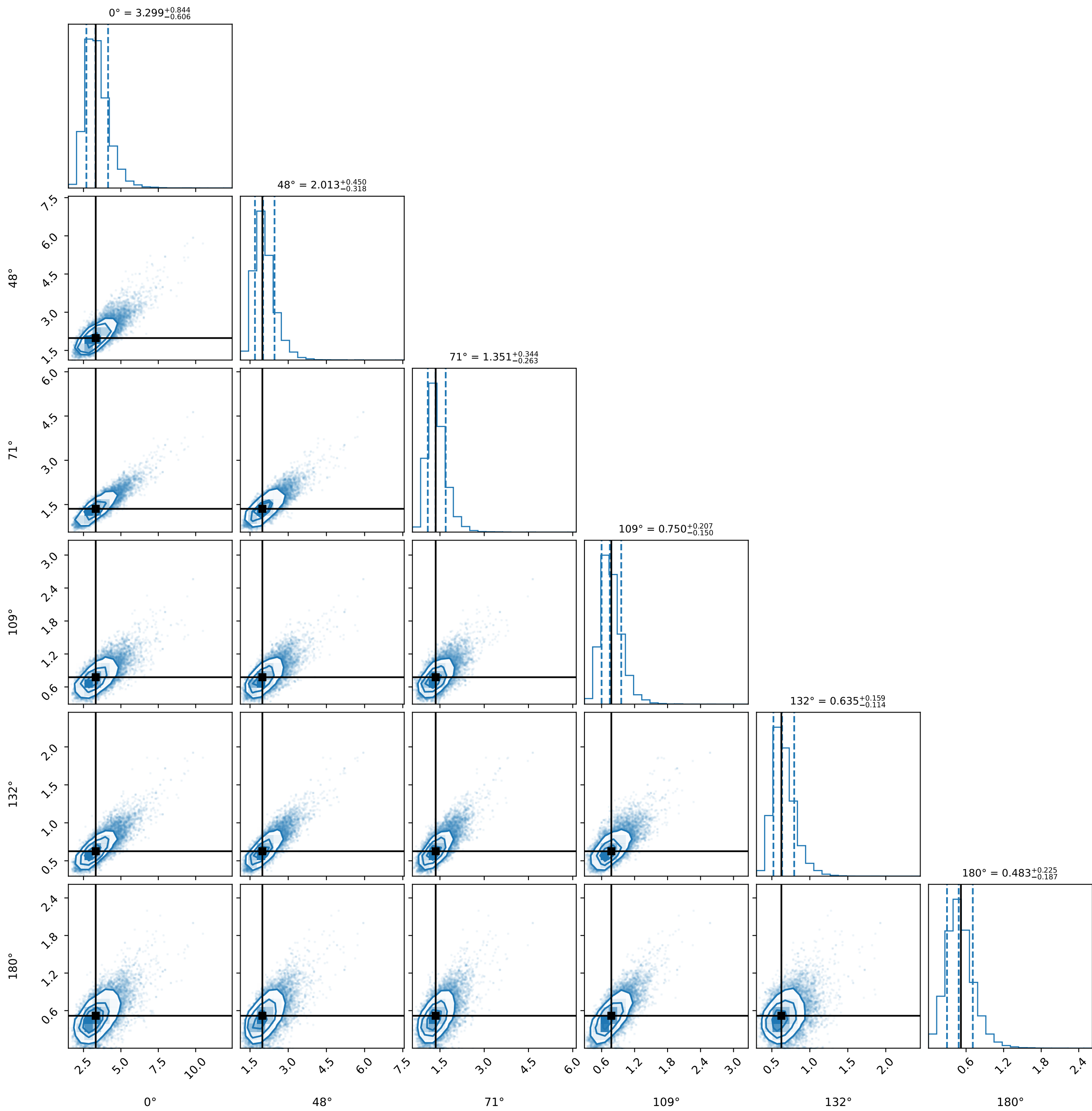
SPF knot posterior ( i = 70^\circ )
