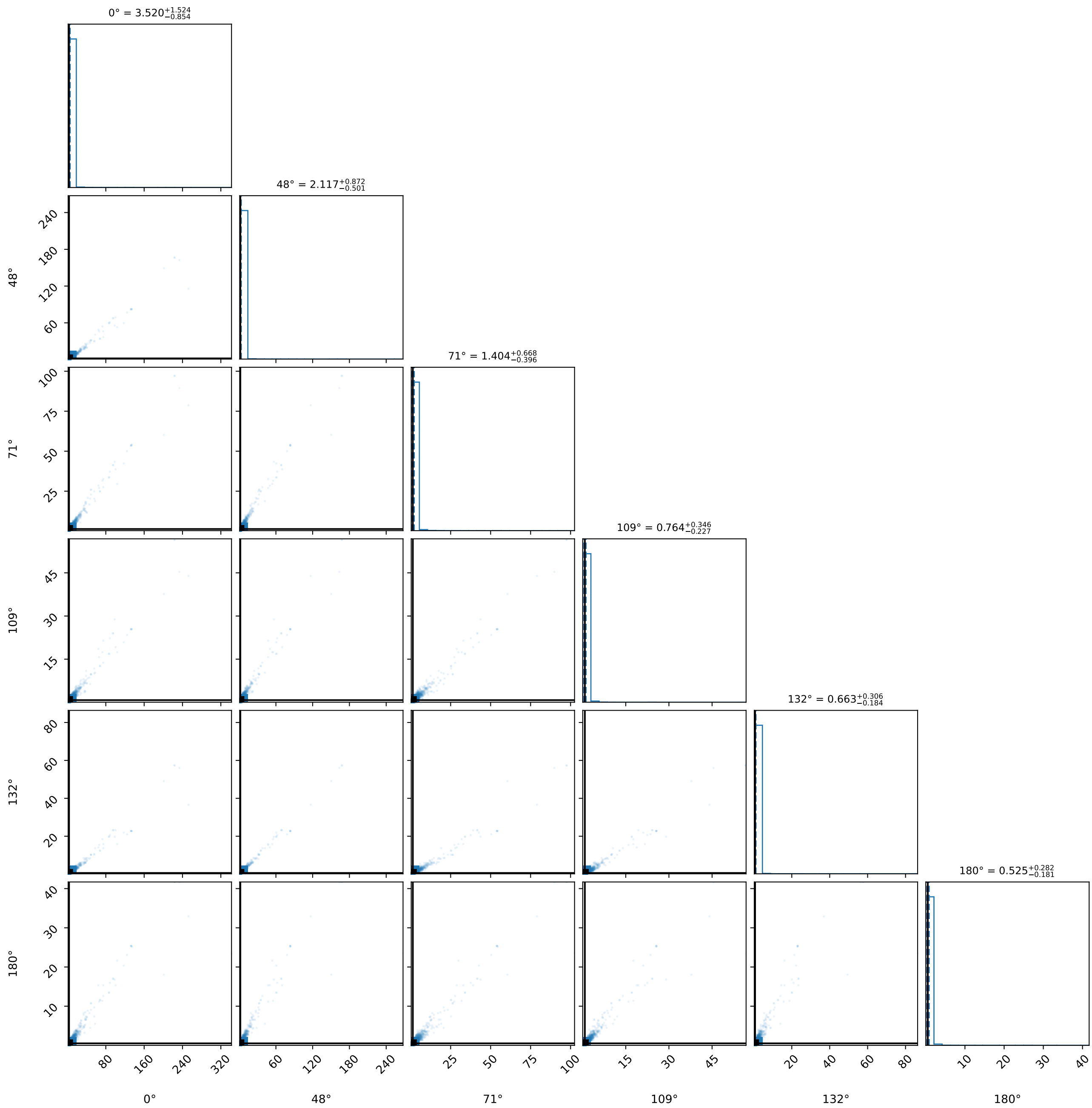
SPF knot posterior ( i = 80^\circ )
