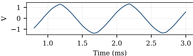
(d) Speaker voltage, full volume: 2.7 V p-p
