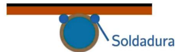
Corte de la unión placa y tubo
