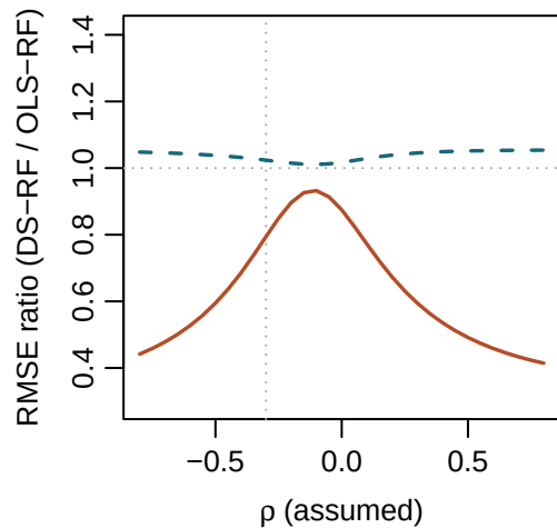
TNIE: \rho_{\text{true}} = -0.3
