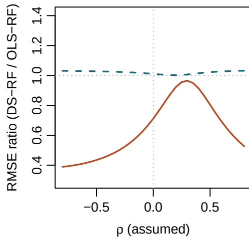
TNIE: \rho_{\text{true}} = 0
