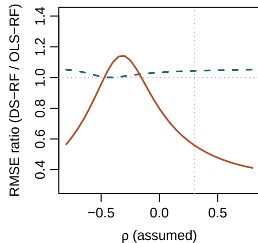
TNIE: \rho_{\text{true}} = 0.3
