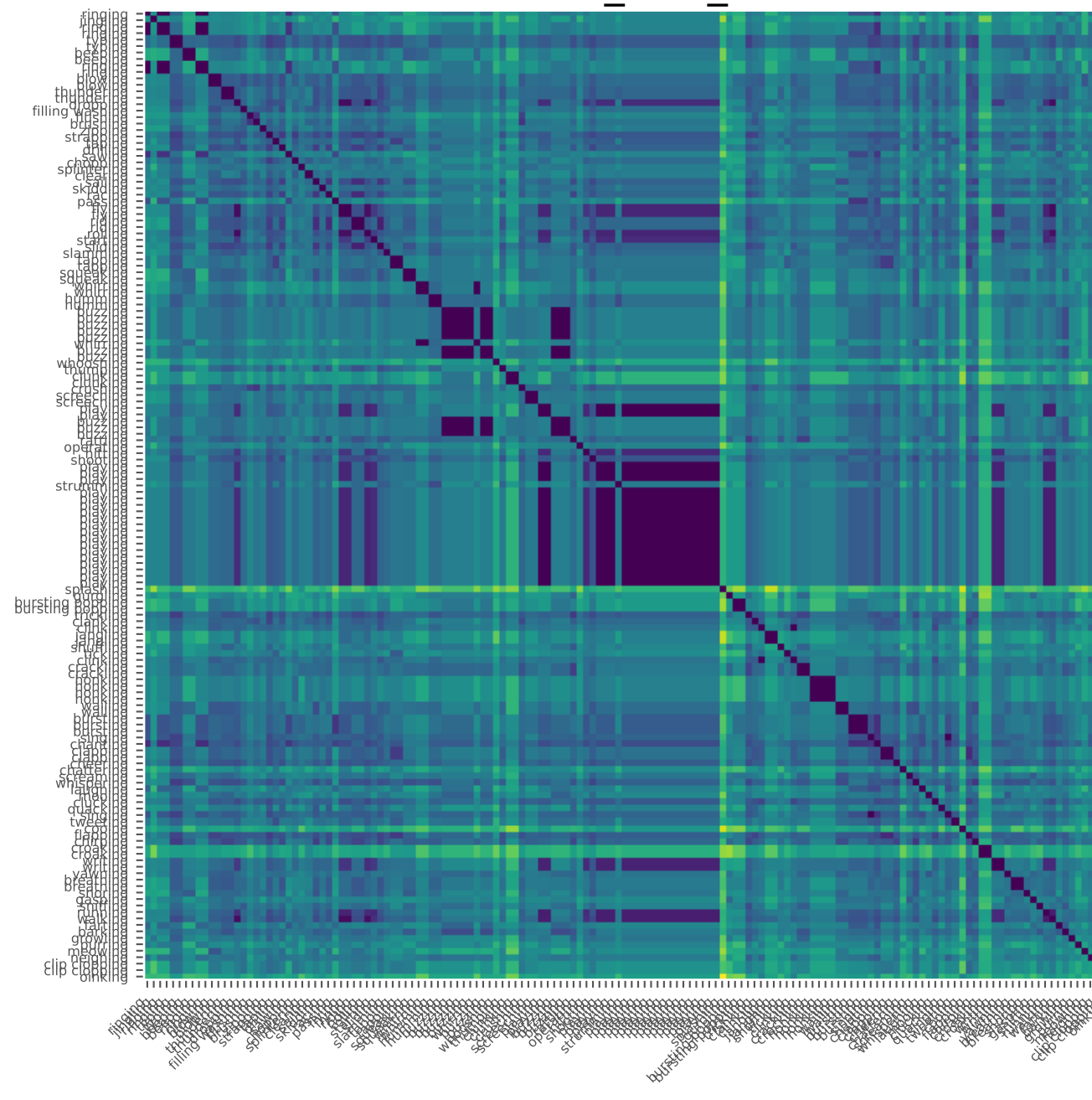
roberta_how_euc
