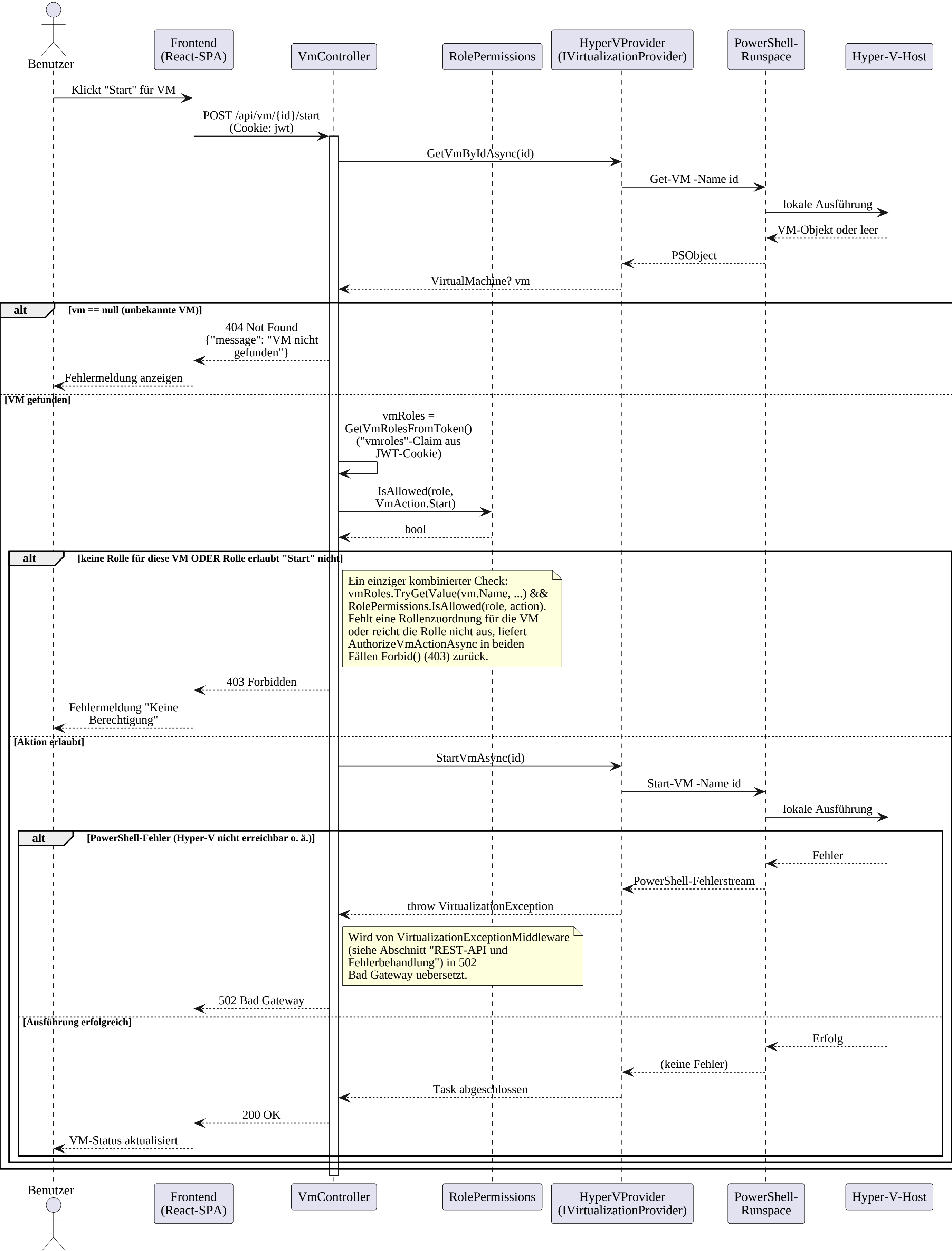
Sequenzdiagramm: VM-Aktion mit Autorisierungsprüfung (Beispiel "Start")
