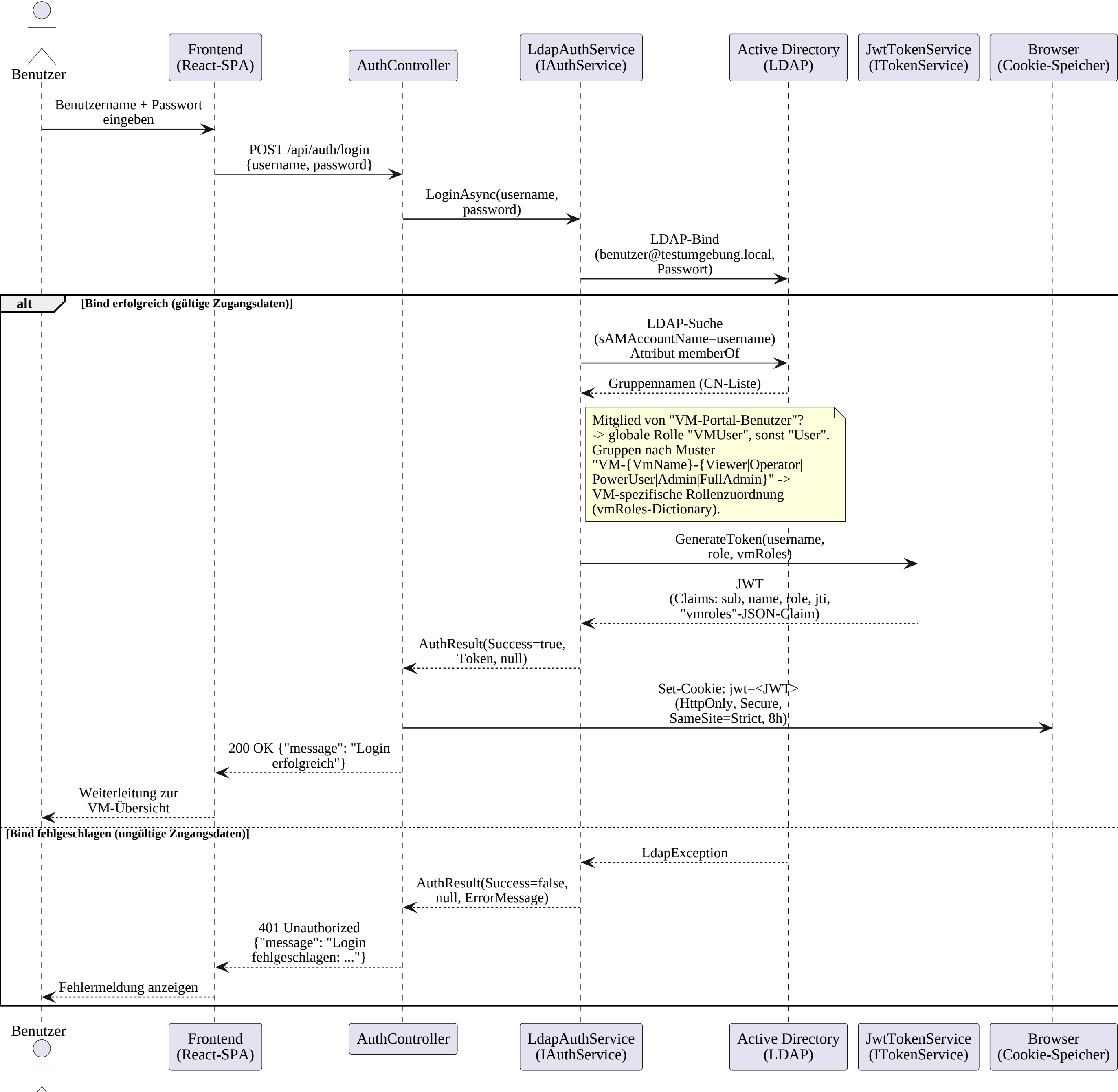
Sequenzdiagramm: Login und Authentifizierung
