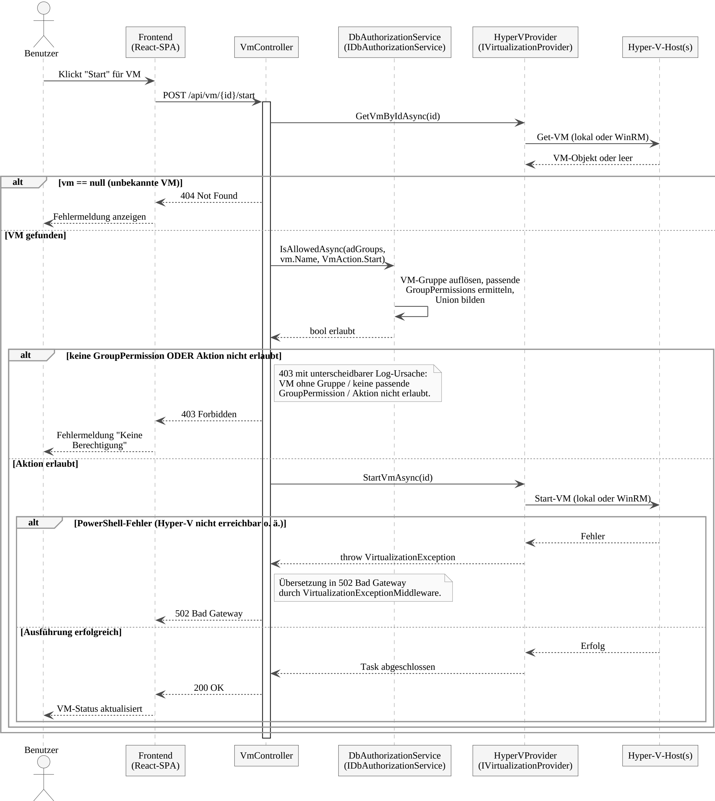
Sequenzdiagramm: VM-Aktion mit Autorisierungsprüfung (Beispiel "Start")
