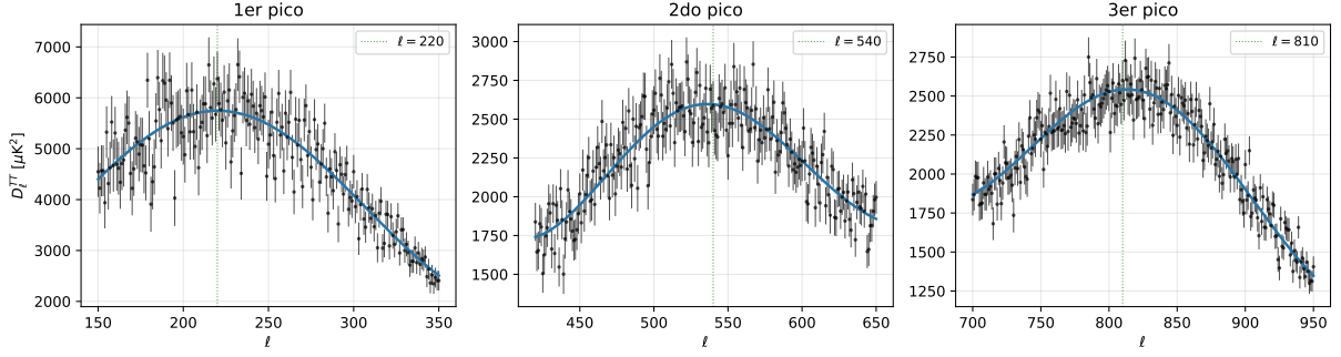
SSEE: Zoom en Picos Acústicos vs Planck 2018
