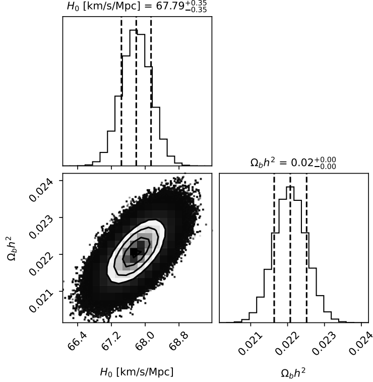
SSEE posterior — MCMC under the H_{\text{alg}} prior (DESI DR2, reframe)
