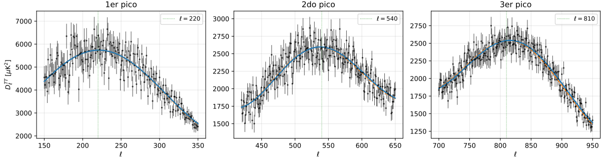
SSEE-V3.6: Zoom en Picos Acústicos vs Planck PR4
