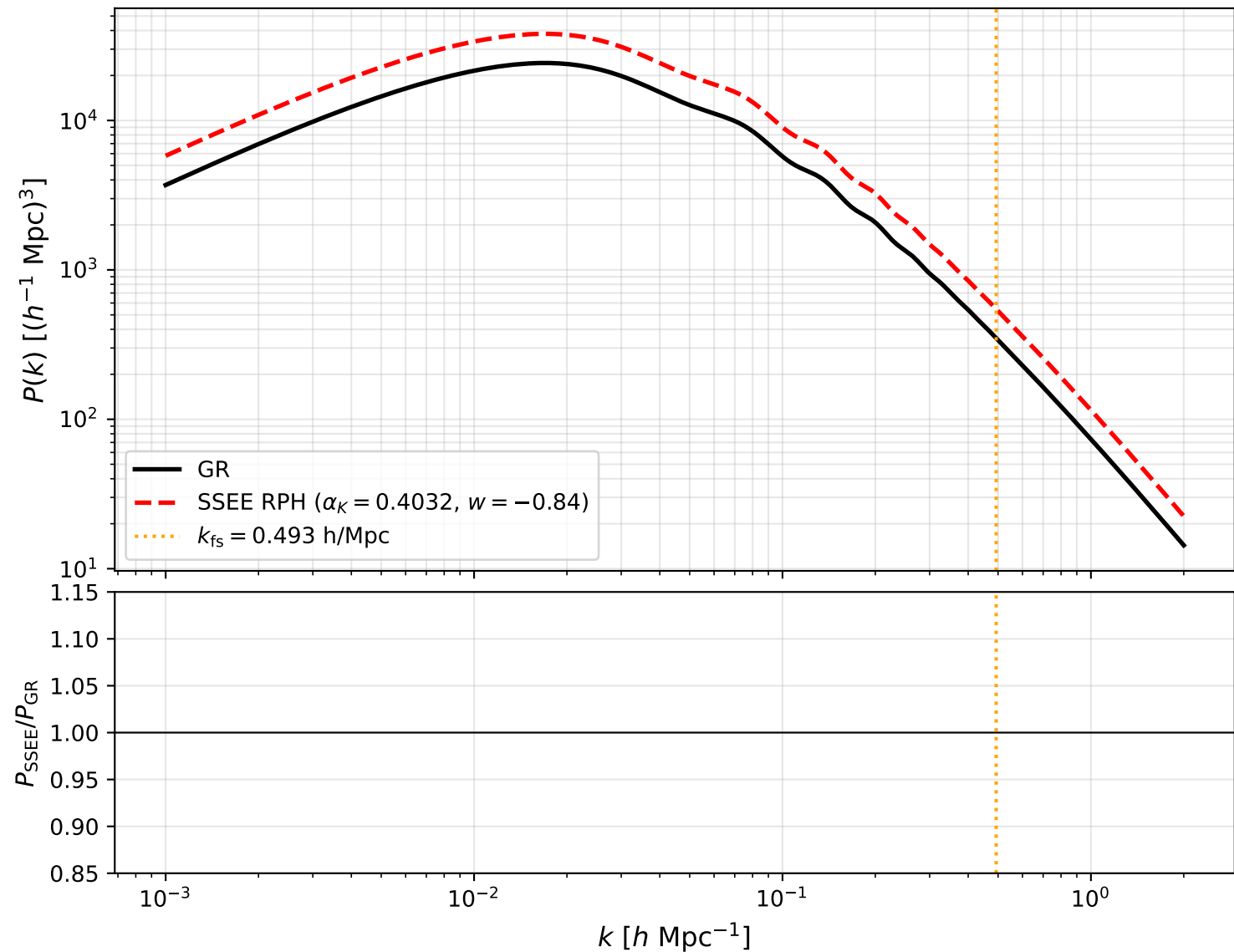
SSEE-V3.6 EFTCAMB — Matter P(k) : EFT kinematicity effect
