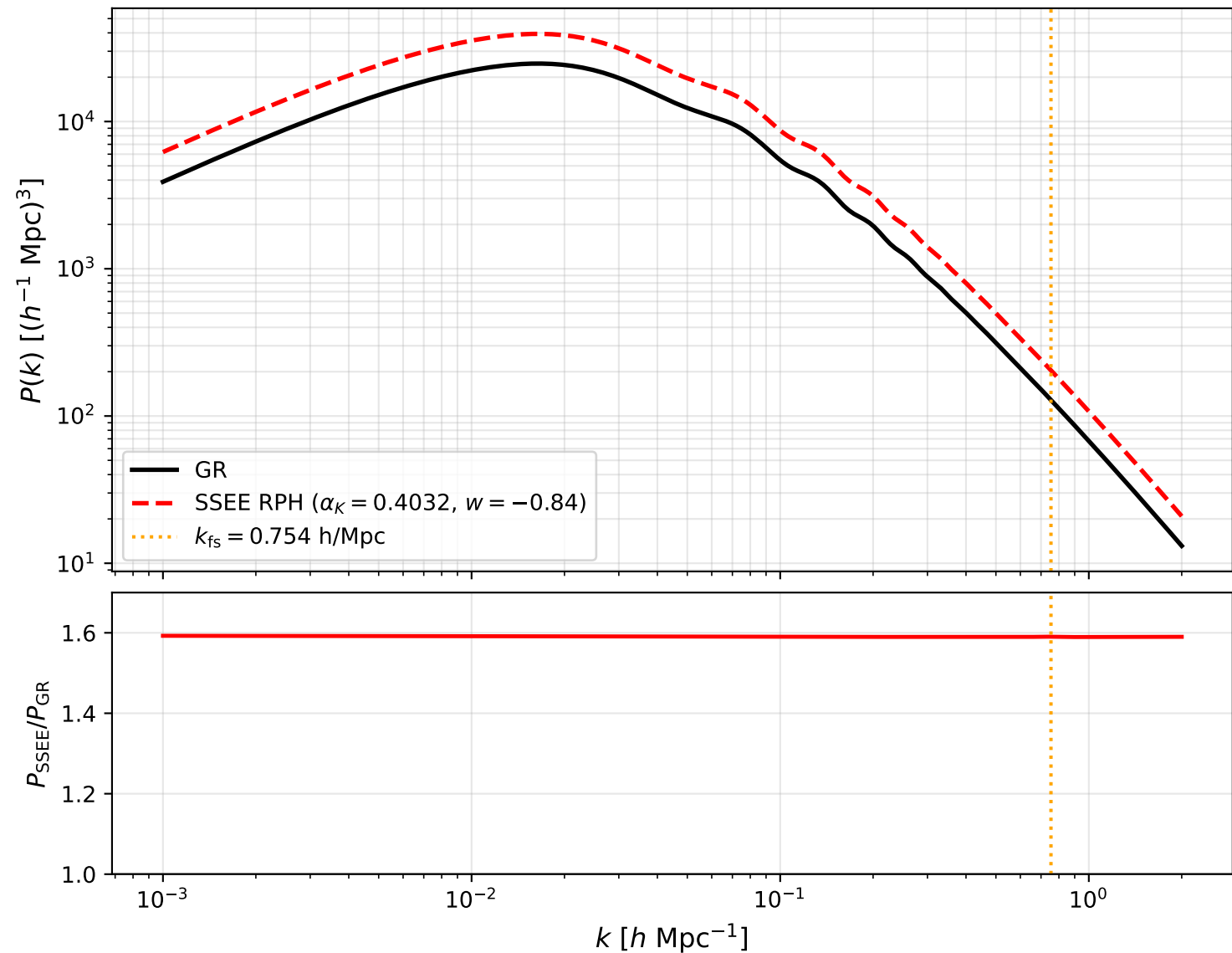
SSEE-V3.6 EFTCAMB — Matter P(k) : EFT kineticity effect
